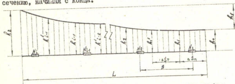
Рис. 2 Схема гидравлического расчета поливного трубопровода с очаговыми увлажнителями конструкции САННИРИ
