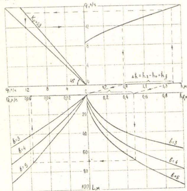
Рис. 4. Номограмма для определения элементов техники полива при очаговом ИО
