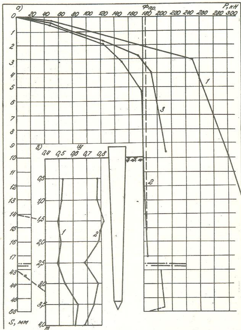
Рис. 3. Графики S=f(H) испытаний несущей способности клиновидной свай: а) 1 - по ускоренной методике без замачивания; 2, 3 - по стандартной и ускоренной методикам в замоченном грунте; б) значения степени влажности грунта G по глубине
