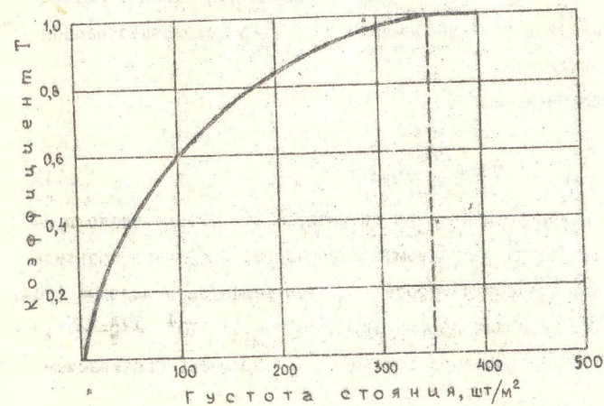
Рис. 5. Коэффициент Т в зависимости от плотности стояния тростника на биоплато
