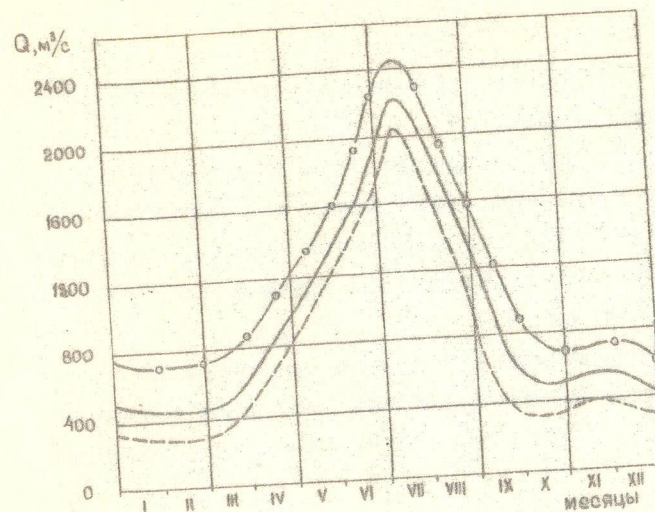
Рис. 1. Изменение осредненного значения расхода воды в створе Туямуви с 1974 по 1984 гг. о — многоточечный ( P = 20\% ), — средний по водности ( P = 50\% ), --- маловодный ( P = 95\% )
