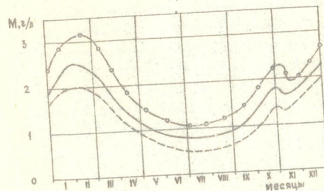
Рис. 2. Прогнозное изменение минерализации воды в Амударье в створе Туямуви о — многоточечный ( P = 20\% ), — средний по водности ( P = 50\% ), --- маловодный ( P = 95\% )
