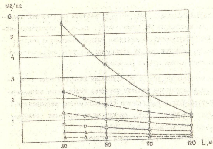
Рис. 4. Изменение концентрации ГХПГ в растениях по длине проточного коллектора \Delta — ГХПГ; \gamma — ГХПГ \bullet — через 2 часа; \circ — через 72 часа; \Delta — через 624 часа
