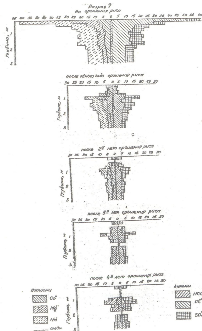
Рис. 2.3. Солевой профиль почвогрунтов и его изменение при орошении культуры риса. ( в м-эвб.)
