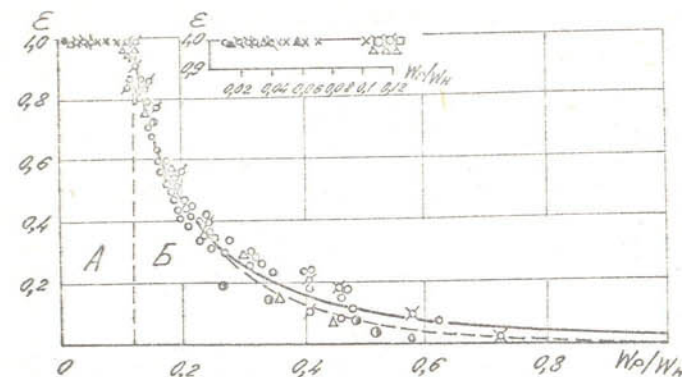
Рис. I. График зависимости степени осветления потока \mathcal{E} и верхних бьефов гидроузлов от отношения W_p/W_H \Delta - фархадский бьеф 1949 г; \bigcirc - то же, 1951 г; \sigma - то же 1952 г; \times - хишрауский бьеф 1958 г; \bigcirc - лабораторные данные (прямолинейный лоток); \bullet - Кайраккумское водохранилище; \blacktriangle - Ташкепринское водохранилище (с 1939 по 1961 г.); \square - Тедженское (1950-1959 гг); \square - Бозсуиский бьеф; \times - лабораторный бьеф 12 I; \phi - Остин новое (США); --- по формуле (2); - - - по формуле (3). I - I зона, Б-II зона
