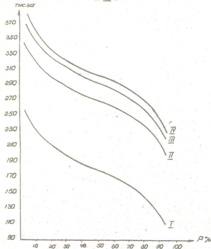
Рис. 6. -График зависимости орошаемых площадей от обеспеченности всех источников орошения: I - при существующем режиме рек; II - при регулировании пятью водохранилищами; III - при использовании коллекторно-сбросных вод; IV - при использовании подземных вод.
