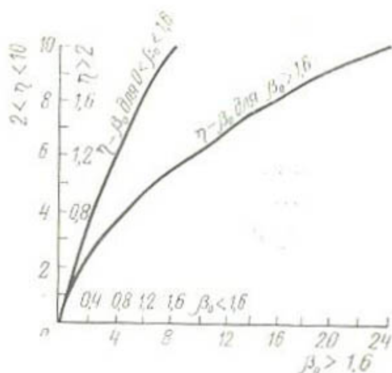
Рис. 23. Зависимость \eta от \beta_0 .
