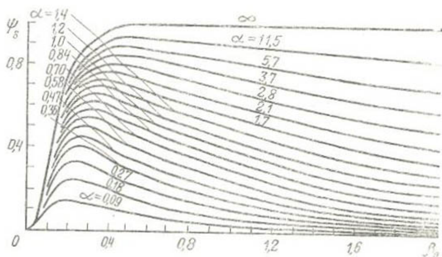
Рис. 39. Зависимость коэффициента притока воды в заполняющиеся водоемы \psi_8 от относительного времени \beta_0 и относительной вместимости водоема \alpha .
