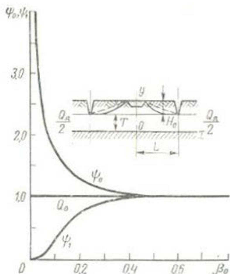
Рис. 32. Зависимость \psi_0 и \psi_1 от \beta_0 при подпертой фильтрации из канала и дренаже.
