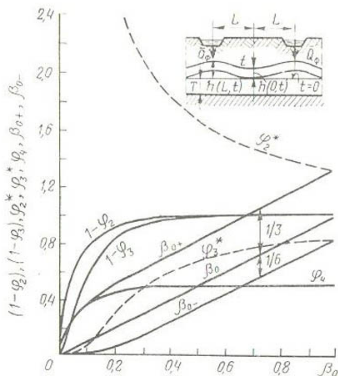
Рис. 30. Зависимости (1-\varphi_2) , (1-\varphi_3) , \varphi_2^* , \varphi_3^* , \varphi_4 , \beta_{0+} , \beta_{0-} от \beta_0 , характеризующие подъем уровня грунтовых вод при неустойчивой свободной фильтрации из системы каналов.
