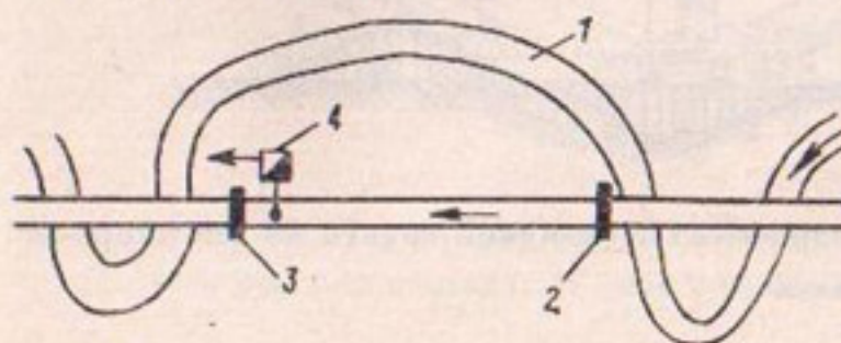
Рис. 27. Спрямление русла водоприемника: 1 — изгиб старого русла; 2, 3 — верхняя и нижняя перемычки; 4 — насосная станция
