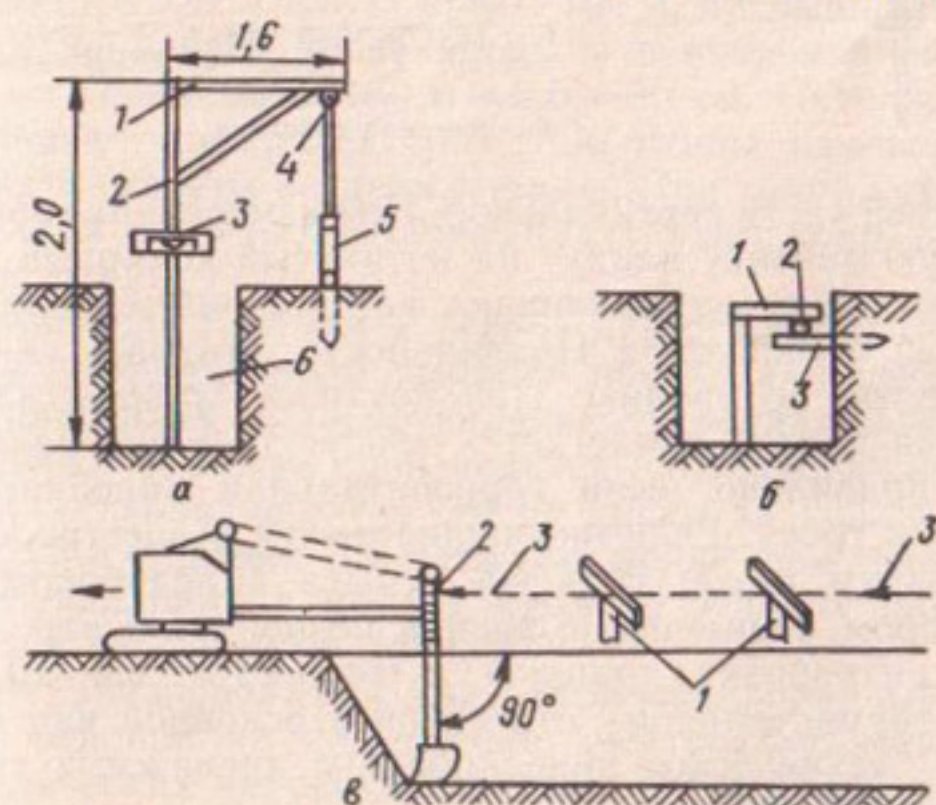
Рис. 60. Способы контроля глубины копания траншей:
