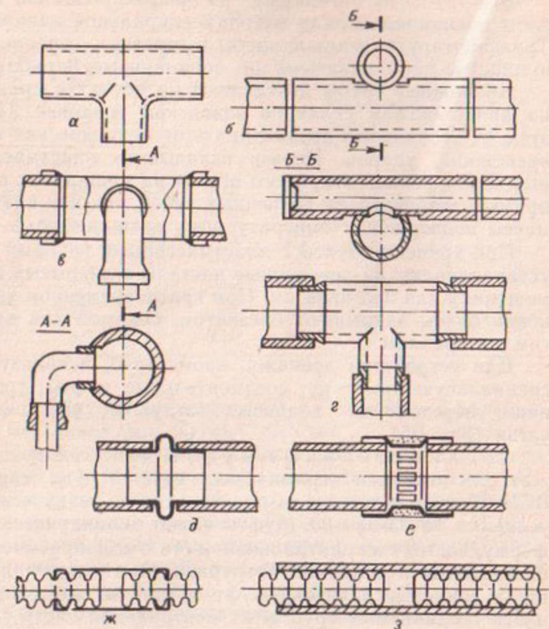
Рис. 25. Дренажная арматура:
