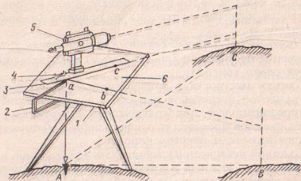
Рис. 7. Мензула:
