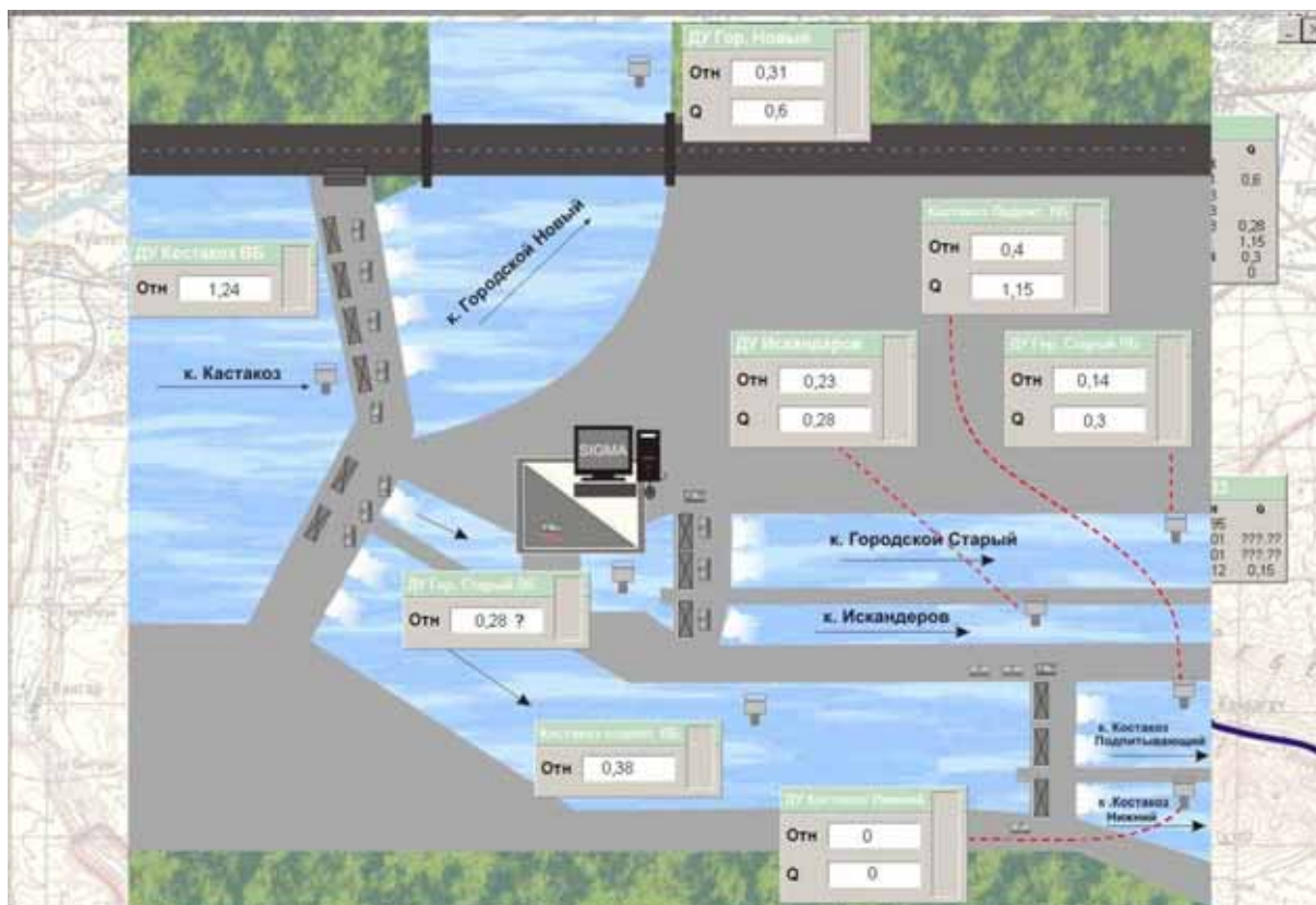
Рис. 19. Узел сооружений Городской на канале Костакоз главная мнемосхема системы SCADA
