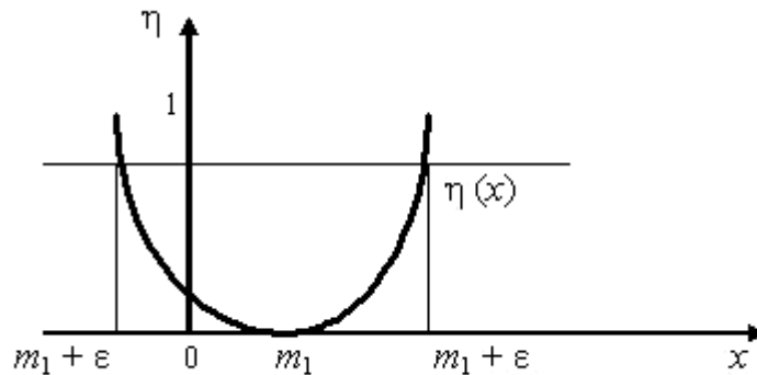
Рисунок 17 – Зависимость длины доверительного интервала от измеряемой величины
