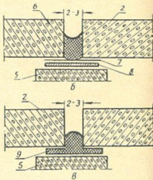
Рис. 12. Уплотнение швов в безраструбных лотках порои́золом, изолюм или битумно-шлаковатной прокладкой:
