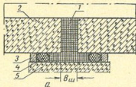
Рис. 12. Уплотнение швов в безраструбных лотках порои́золом, изолюм или битумно-шлаковатной прокладкой:
