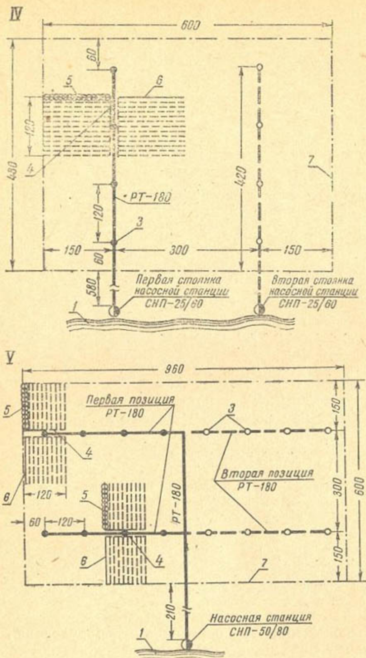
Рис. 7. Схемы орошения участков с помощью установок КДУ-55М: I — площадь орошения за сезон 25,2 га; II—IV — 28,8 га; V — 57,6 га; 1 — водосточник; 2 — подводящая часть трубопровода; 3 — труба-гидрант РТ-180X125; 4 — вспомогательный трубопровод; 5 — первое крыло; 6 — второе крыло; 7 — граница орошаемой площади.
