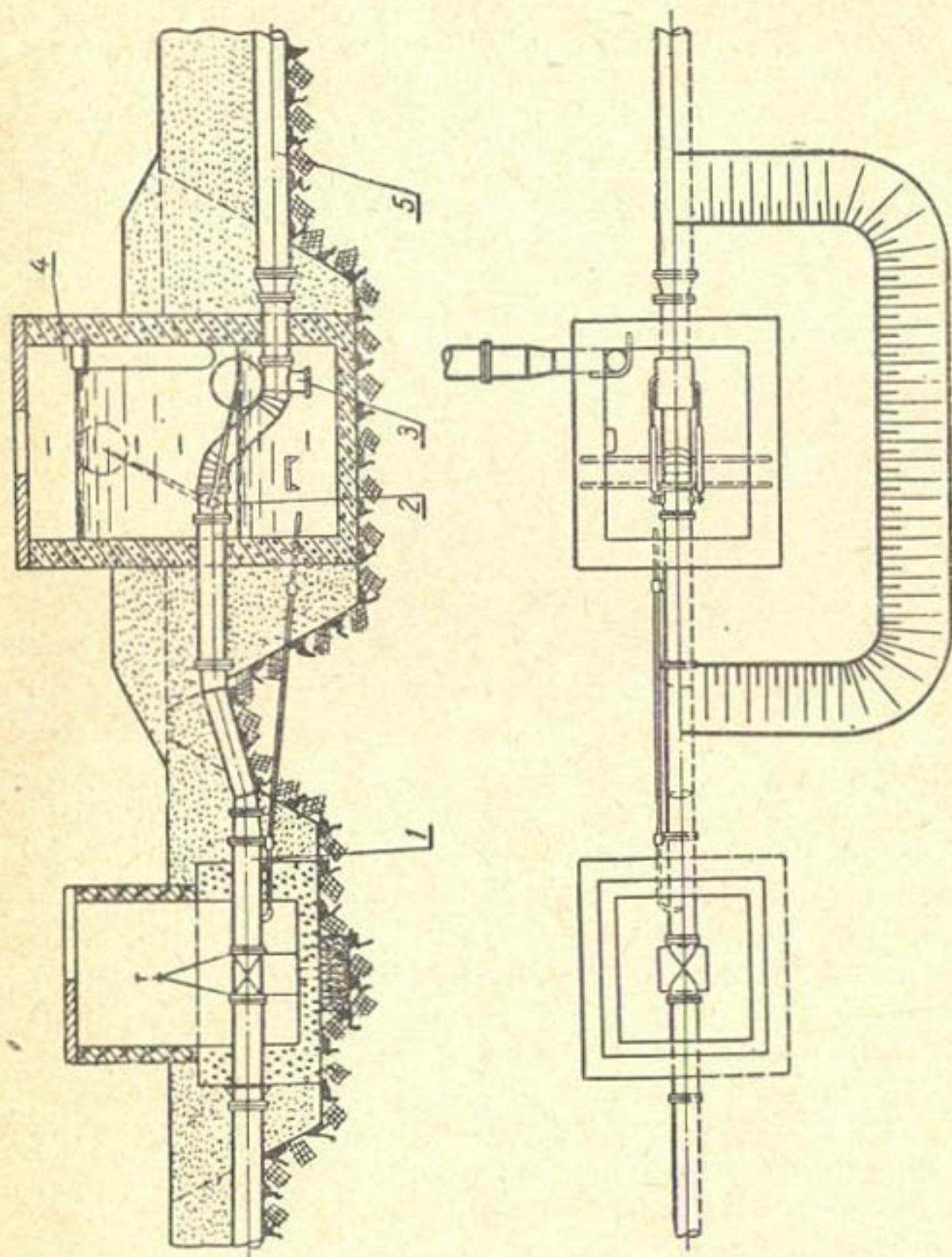
Рис. 67. Гаситель напора с патрубком-отводом: 1 — вышерасположенный трубопровод; 2 — дроссельный клапан; 3 — патрубок-отвод; 4 — ко- лodeц; 5 — нижерасположенный трубопровод.
