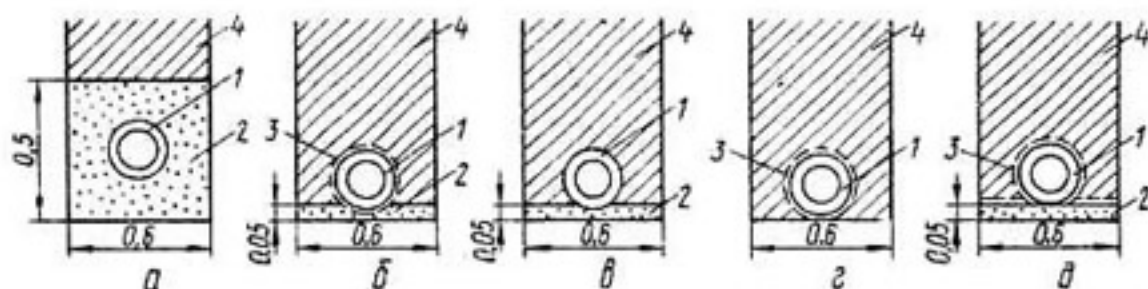
Рис. 40. Варианты конструкций дренажа из пористо-бетонных трубофильтров при устройстве траншей дрепоукладчиком типа Д-659А:
