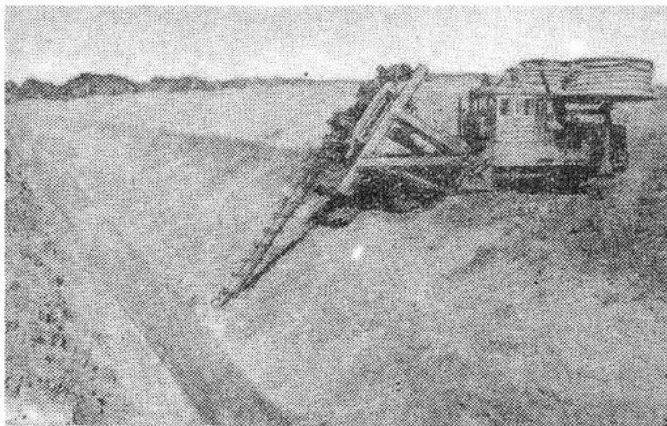
Рис. 39. Шнековый дрепоукладчик БШУ-4, разрабатываемый НИИСПом Госстроя СССР (Ингулецкая оросительная система, Николаевская область, июнь 1974 г.).
