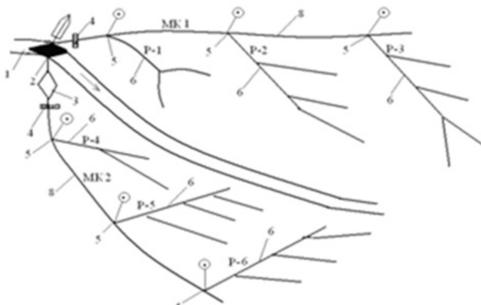
Рисунок 1.6 – Линейная схема ирригационной системы с двухсторонним командованием: 1 – река; 2 – водозаборное сооружение; 3 – отстойник; 4 – гидросты; 5 – водовыпуски; 6 – распределительные каналы; 7 – дюкер; 8 – магистральный канал
