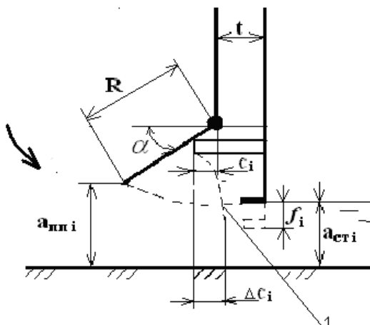
Рисунок 2.34 – Расчетная схема нижнего узла усовершенствованного стабилизатора расхода: 1 – траектория перемещения концевой участка штанги взаимодействия при перемещении плоского затвора; \Delta c – необходимая величина смещения штанги взаимодействия при закрытии затвора
