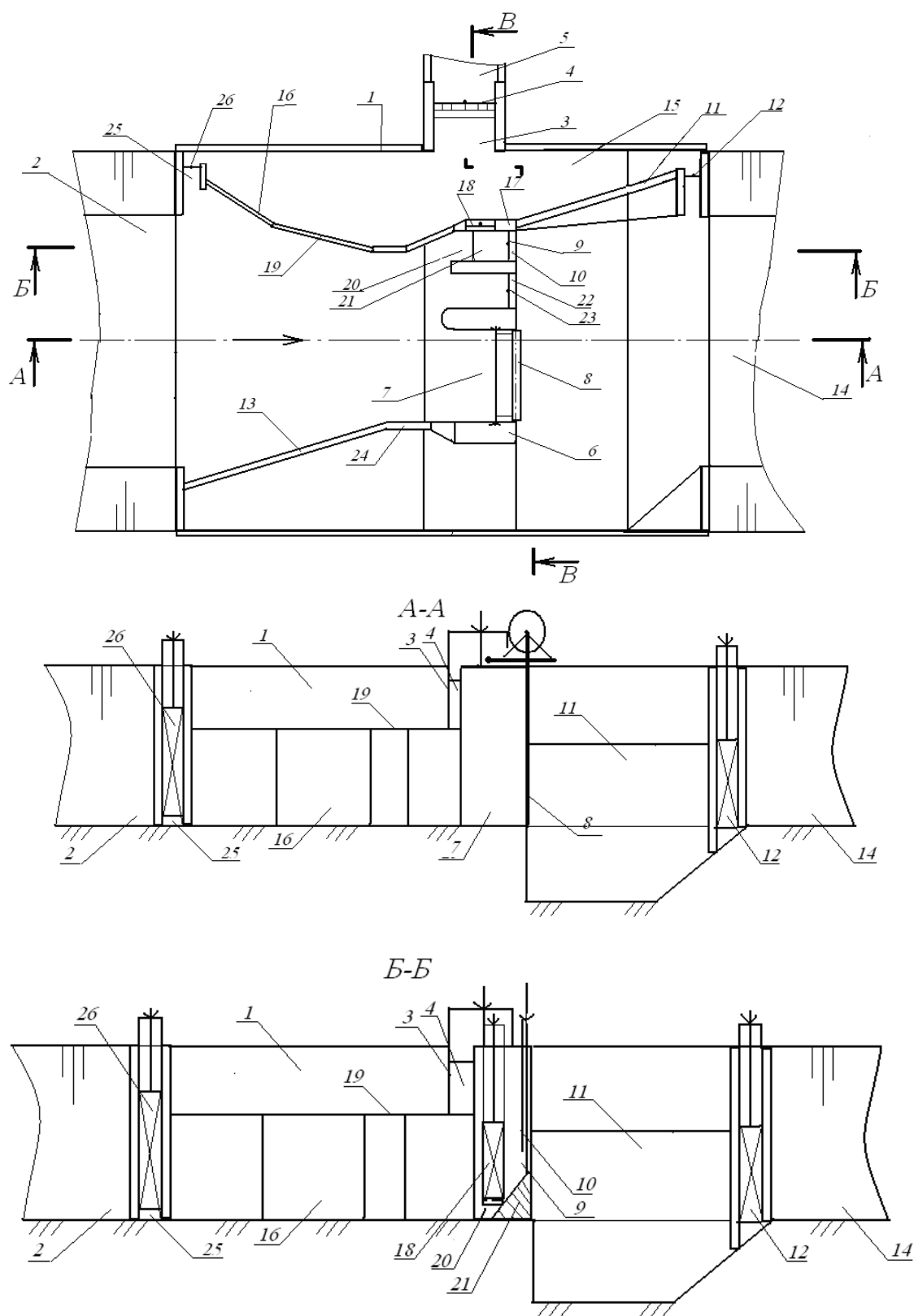
Рисунок 2.29 – Компоновочная схема ВСДГ-2: 1 – береговой устой; 2 – подводящее русло; 3 – водоприемный оголовок; 4 – стабилизатор расхода; 5 – отводящий канал; 6 – подпорное сооружение; 7 – речной пролет; 8 – авторегулятор уровня верхнего бьефа; 9 – затвор; 10 – промывное отверстие; 11 – автоводослив; 12 – затвор сбросного отверстия; 13 – автоводослив; 14 – отводящее русло; 15 – водоприемная камера; 16 – ломаный в плане четырехсекционный порог; 17 – разделительный бычок; 18 – зимнее отверстие, прикрываемое затвором; 19 – горизонтальный гребень порога; 20 – промывной тракт; 21 – донная вставка; 22 – отверстие дополнительного промывного тракта; 23 – сдвоенный затвор; 24 – концевая секция автоводослива; 25 – верхнее водоприемное отверстие; 26 – плоский затвор
