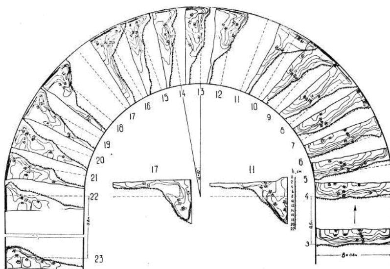
Рисунок 2.6 – Распределение продольных составляющих скоростей на повороте русла с размываемым дном
