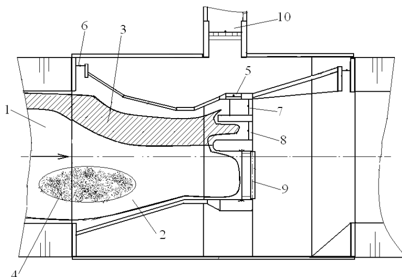
Рисунок 4.23 – Схема размещения призмы наносов в верхнем бьефе водозаборного сооружения при подаче по подводному руслу расхода двухфазного потока жидкости (вода – наносы) Q_{75\%} малой горной реки с коэффициентом водозабора 0,9: 1 – подводное зарегулированное русло; 2 – призма наносов; 3 – зона промывки; 4 – зона максимальной высоты призмы наносов; 5 – отверстие зимнего водозабора; 6 – верхнее водоприемное отверстие; 7 – промывное отверстие, перекрываемое затвором; 8 – отверстие дополнительного промывного тракта, перекрываемое двойным затвором; 9 – затвор речного пролета; 10 – отводящий канал
