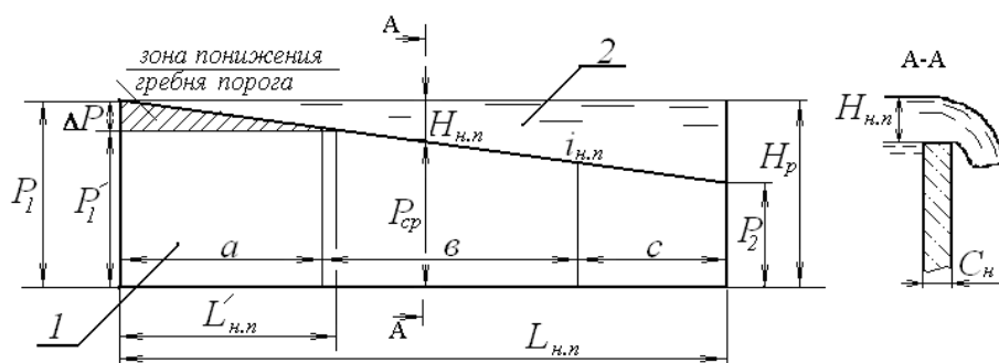
Рисунок 4.4 – Расчетная схема ломаного в плане наносозащитного порога: 1 – наносозащитный порог; 2 – водосливной фронт при истечении через гребень наносозащитного порога; P_1' – высота порога в начале после понижения; L_n – длина области понижения порога
