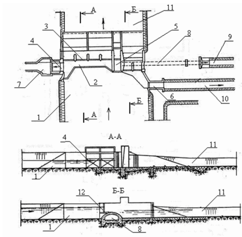
Рисунок 1.13 – Компоновочная схема сооружения европейского типа с боковыми водоприемниками: 1 – подводящее русло; 2 – понур; 3 – речные пролеты плотины, перекрытые затворами; 4 – боковой водоприемник левобережного канала; 5 – бычковый водоприемник правобережного канала; 6 – боковой водоприемник деривационного канала межколхозной ГЭС; 7 – левобережный канал; 8 – гусек; 9 – правобережный канал; 10 – деривационный канал; 11 – отводящее русло; 12 – водосливная стенка
