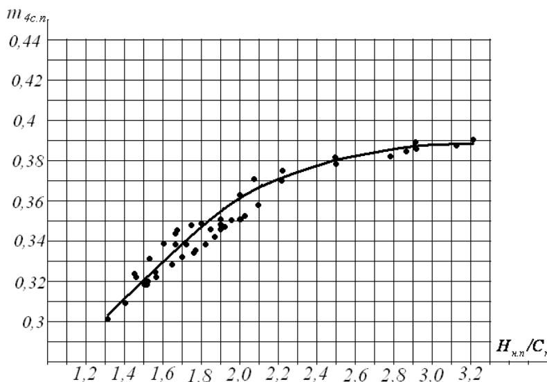
Рисунок 4.13 – Зависимость коэффициента расхода четырехсекционного ломаного в плане порога m_{4c.n} от относительного напора над гребнем порога H_{н.п} / C_{н.п}
