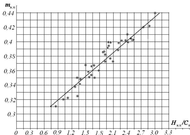
Рисунок 4.2 – График зависимости коэффициента расхода трехсекционного ломаного в плане наносозащитного порога от отношения напора воды над гребнем порога H_{n,n} к ширине порога в поперечном сечении C_n
