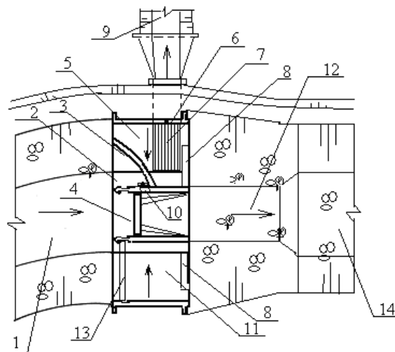
Рисунок 1.27 – Водозаборное сооружение Тяньшаньского типа: 1 – подводящее русло; 2 – понур; 3 – косо направленный порог; 4 – речной пролет; 5 – водоприемная камера; 6 – водоприемник; 7 – сороудерживающая решетка; 8 – автоводосливы; 9 – отводящий канал; 10 – промывное отверстие; 11 – аванкамера; 12 – колодец; 13 – ремонтный затвор; 14 – отводящее русло
