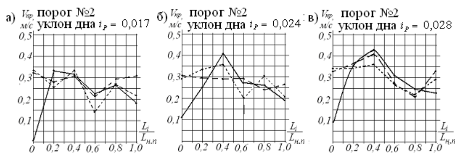
Рисунок 4.15 – Зависимости изменения абсолютных величин продольных составляющих результирующих скоростей воды в циркуляционном вальце по длине четырехсекционных порогов V_{пр} = f(L_i/L) при устройстве донной вставки
