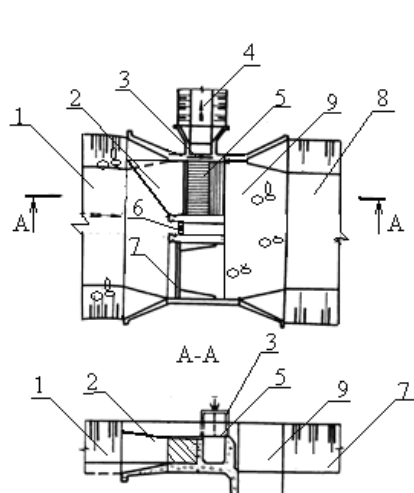
Рисунок 1.26 – Водозаборное сооружение Киргизского типа: 1 – подводящее русло; 2 – донный порог; 3 – регулятор расхода; 4 – отводящий канал; 5 – решетка, перекрывающая водоприемную галерею; 6 – промывник открытого типа; 7 – речной пролет; 8 – отводящее русло; 9 – водобойный колодец
