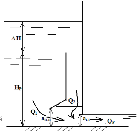
Рисунок 2.33 – Расчетная схема стабилизатора расхода с поворотной пластиной
