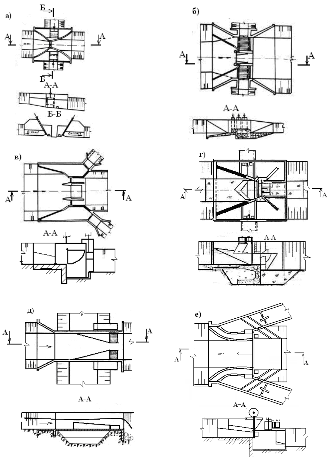
Рисунок 1.29 – Компоновочные схемы водозаборных гидроузлов с двухсторонним водоотбором: а – водозабор Я.В. Бочкарева и А.С. Лугового, б, в – водозаборы по схеме Г.В. Соболина; г – схема водозабора, предложенная Г.В. Соболиным и А.И. Рохманом, д – схема водозабора К.Ф. Артамонова и С.С. Сатаркулова; е – водозабор Б.И. Мельникова с двойным наносозащитным порогом
