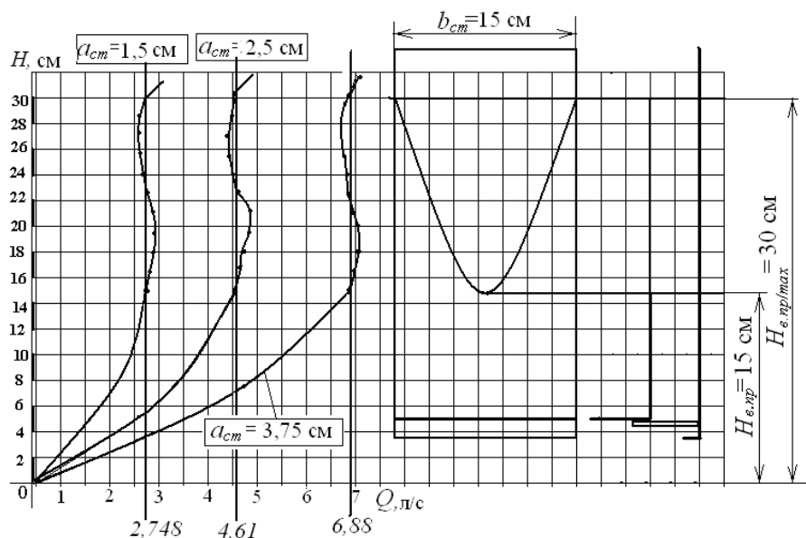
Рисунок 4.19 – Совмещенная расчетная схема стабилизатора расхода и графика зависимости Q=f(H_{\text{вк}})
