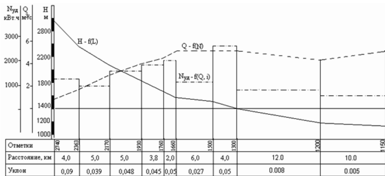
Рисунок 1.9 – Характерный продольный профиль малых горных рек Кыргызстана
