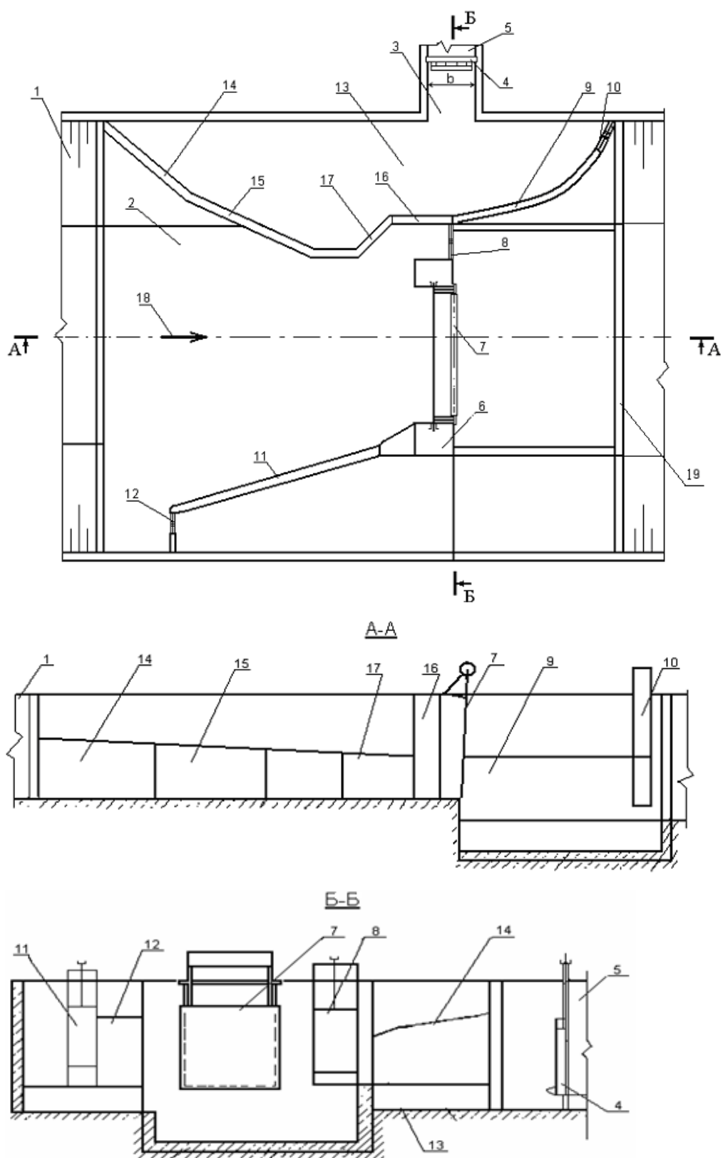
Рисунок 2.28 – Компановочная схема (ВСГР (Патент КР № 920): 1 – береговой устой, 2 – подводящее русло, 3 – водоприемный оголовок, 4 – стабилизатор расхода, 5 – отводящий канал, 6 – подпорное сооружение, 7 – речной пролет, 8 – затвор промывного отверстия, 9 – криволинейный в плане автоводослив, 10 – затвор сбросного отверстия, 11 – автоводослив, 12 – затвор наносоотводящего отверстия, 13 – водоприемная камера, 14 – ломаный в плане четырехсекционный порог, 15 – концевая часть наносозащитного порога, выступающая в сторону речного пролета, 16 – разделительный бычок, 17 – концевая секция порога, 18 – динамическая ось потока в верхнем бьефе, 19 – отводящее русло
