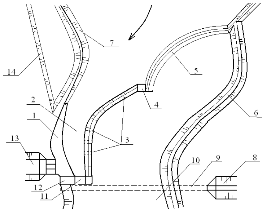
Рисунок 1.16 – Ферганский тип водозаборного гидроузла с криволинейным карманом: 1 – криволинейный Г-образный наносозащитный порог; 3 – донные трубы; 4 – шлюз; 5 – водослив; 6 – левобережная дамба; 7 – правобережная дамба; 8 – левобережный канал; 9 – дюкер; 10 – отводящее русло; 11 – промывник; 12 – водозабор дюкера; 13 – водозабор правобережного канала; 14 – коренной берег
