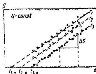
Рис. 69. График временного понижения уровня S=f(t) .
