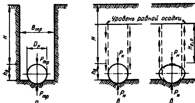
Рис. 13. Расчетные схемы нагрузок на трубы:
