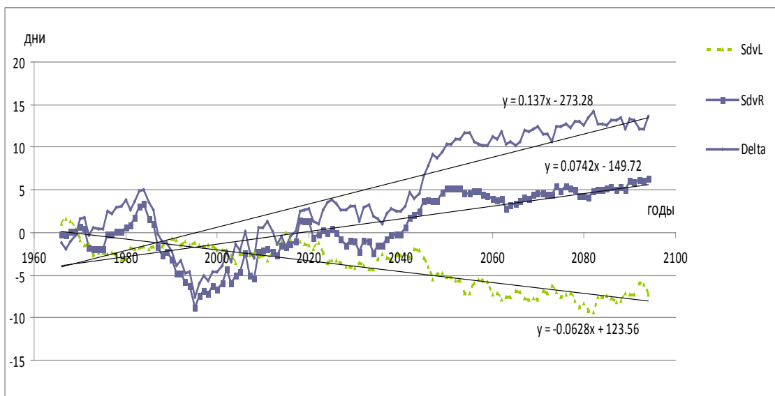
Рис. 24. Ожидаемые изменения дат устойчивого перехода через 5 °C
