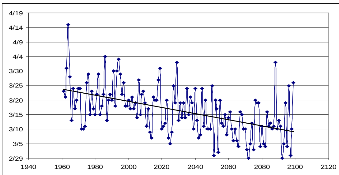
Рис. 23. Изменение дат устойчивых переходов через 10 °C
