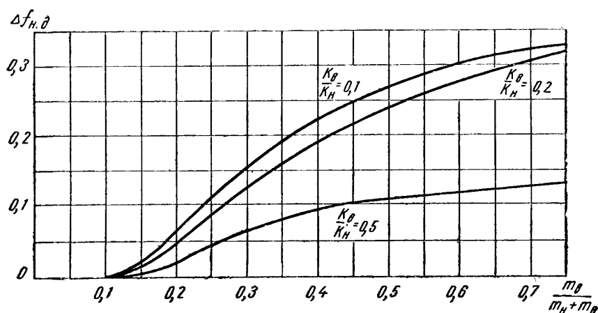
Рис. 44. График определения величины \Delta f_{н.д} ( \Delta f_{н.д} = 0 при \frac{k_b}{k_n} = 1 )
