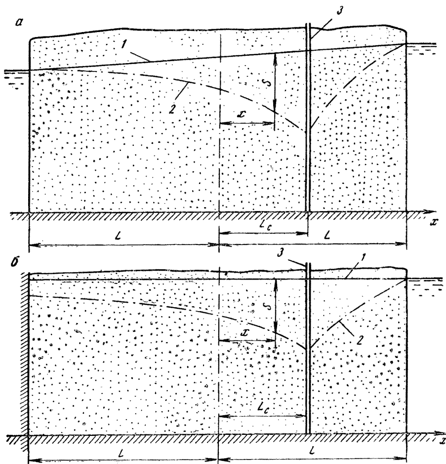
Рис. 60. Схемы к расчету ряда скважин в полосовом пласте: a — пласт между областями питания — стока, б — пласт между областью питания — стока и непроницаемым контуром; 1 — кривая депрессии естественного потока; 2 — то же при откачке из скважины; 3 — линия скважин
