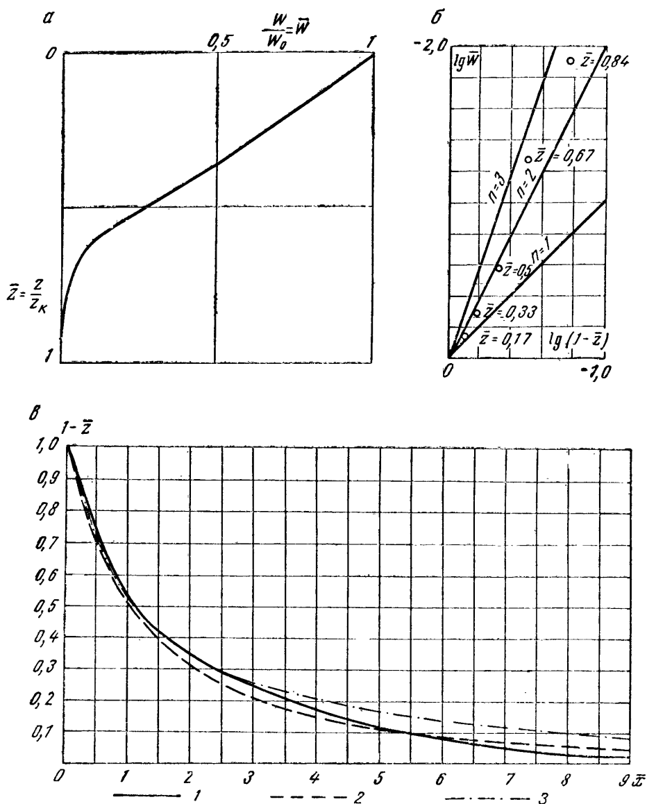
Рис. 16. Данные примера расчета фильтрационного потока с испарением, зависящим от глубины грунтовых вод:
