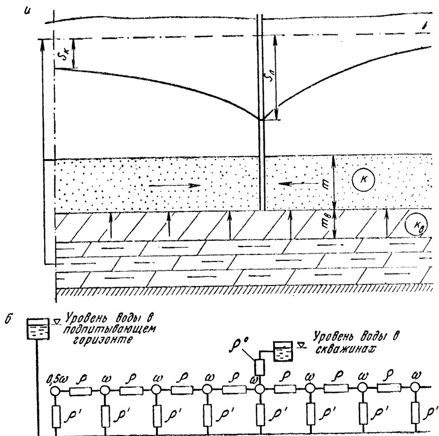
Рис. 69. Моделирование фильтрации при подпитывании из горизонта с постоянным напором: а — фильтрационная схема, б — схема гидромодели
