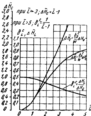
Рис. 66. Графики зависимостей \Delta \bar{H}_c , \Delta \bar{H}_L , \delta_L^c от \bar{L} = b_0 L
