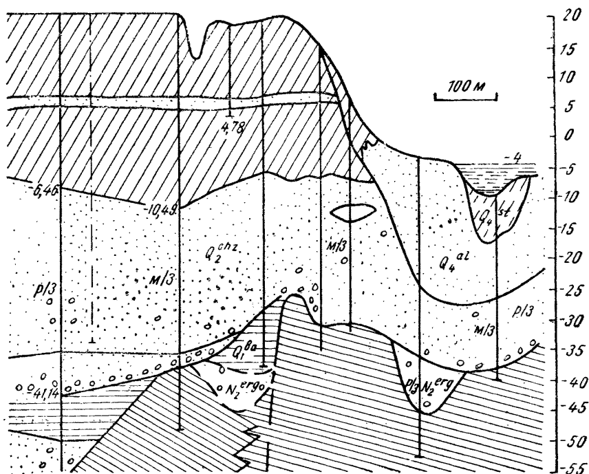
Рис. 24. Данные для определения параметров по створу Гидропроекта у г. Волгограда (левый берег р. Волги): а — план расположения скважин, б — графики колебания уровней водоносного горизонта в наблюдательных скважинах (по данным Гидропроекта), в — разрез по створу Гидропроекта
