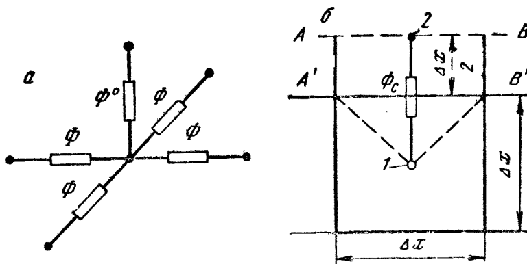
Рис. 58. Схема сетки у блока со скважиной: а — сетка сопротивлений; б — схема блока со скважиной; 1 — скважина, 2 — центр соседнего блока
