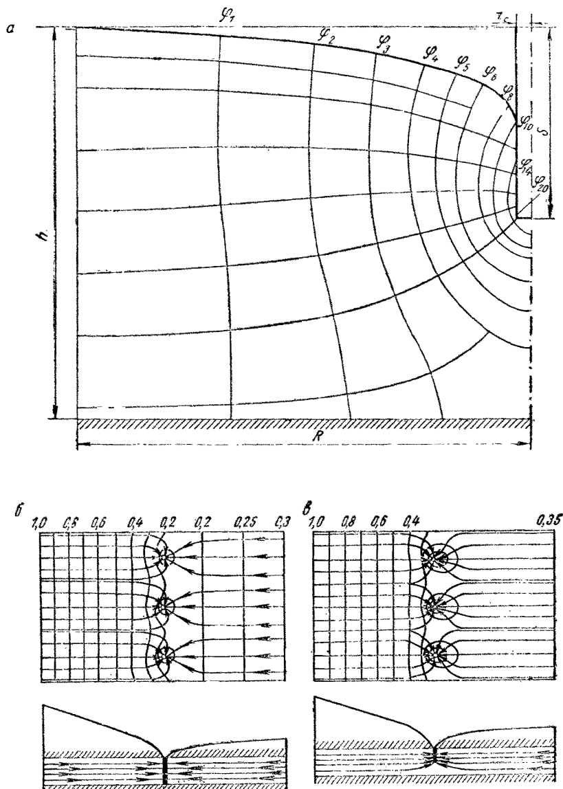
Рис. 31. Сетка потока вблизи скважин: а — одиночная несовершенная скважина в безнапорном потоке, по Наргангу (Nahrgang G.), [45]; б, в — поток к цепочке совершенных и несовершенных скважин в полосе между двумя областями питания, по С. К. Абрамову [1]
