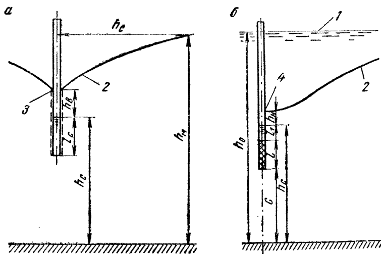
Рис. 33. Схема несовершенных скважин: а — с незатопленным фильтром, б — с затопленным фильтром; 1 — статический уровень воды, 2 — кривая депрессии при работе скважин, 3 — точка высачивания, 4 — точка наивисания
