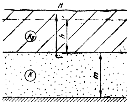
Рис. 18. Схема двухслойной среды
