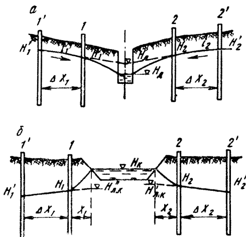
Рис. 49. Наблюдательные створы для определения сопротивлений на несовершенство: а — дрен, б — канала
