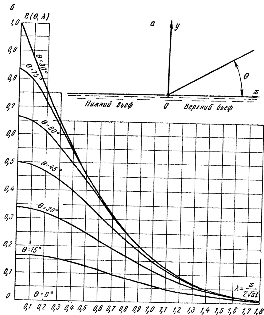
Рис. 13. К расчету обходного потока на плоскости при точечном примыкании сооружения:
