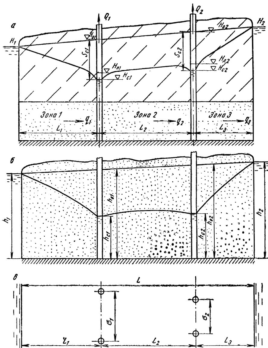
Рис. 53. Два ряда скважин между двумя областями питания или стока: a , б — разрезы для напорного и однородного безнапорного потоков, в — план расположения скважин
