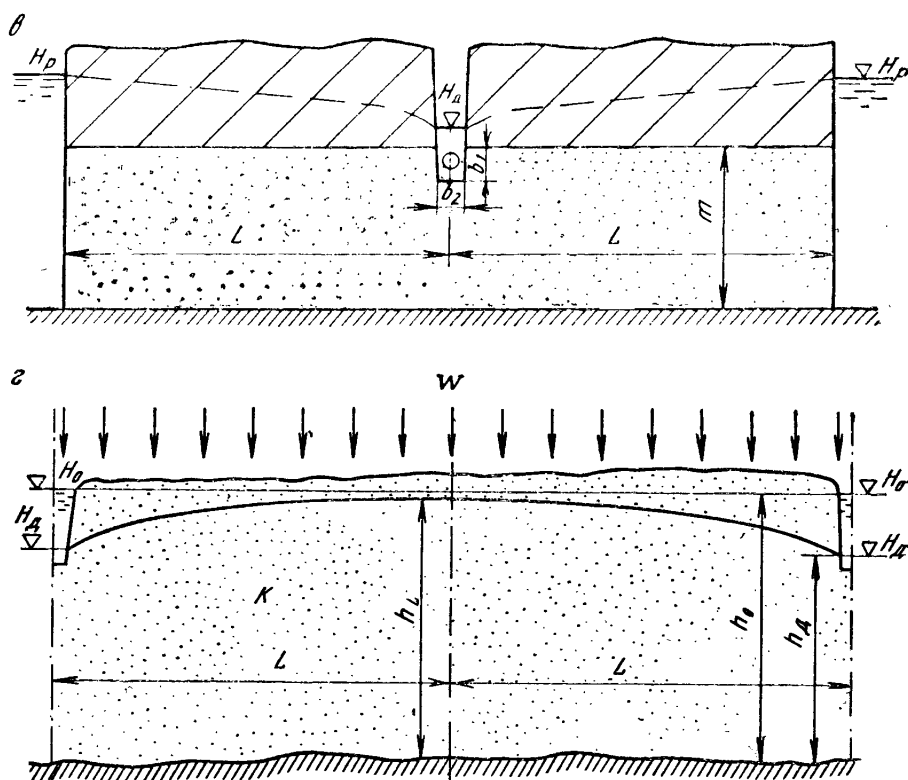
Рис. 39. Схема расположения горизонтальных дрен: а, б — при одностороннем притоке, в — при двухстороннем симметричном притоке; з — в междуречном массиве
