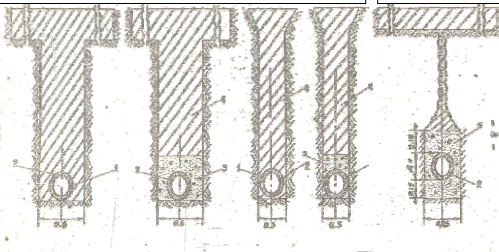
Рис. 1. Дрены из пластмассовых труб с искусственными и комбинированными ЗФМ: 1 – пластмассовая труба, 2 – искусственный ЗФМ, 3 - обсыпка некондиционированными песчано-гравийными смесями, 3 – грунт обратной засыпки.
