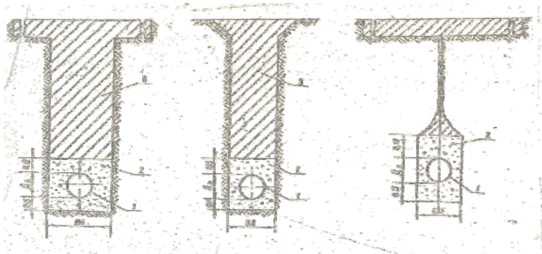
Рис. 1. Дрены из пластмассовых труб: 1 – пластмассовая труба, 2 – обсыпка песчано-гравийной смесью, 3 – грунт обратной засыпки.
