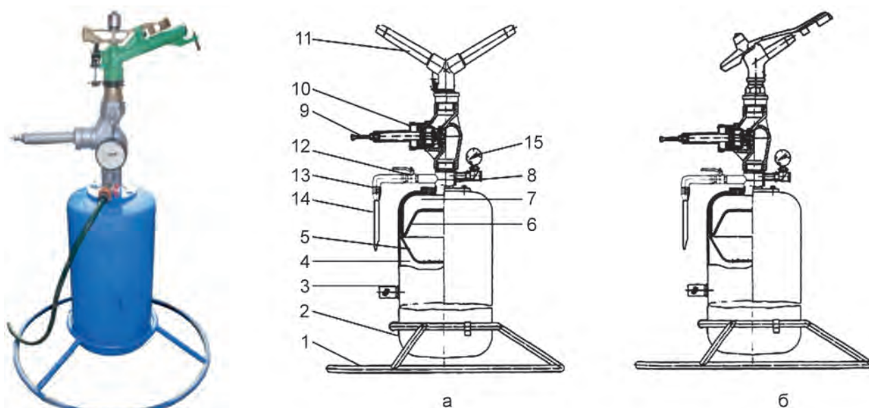
Рис. 6.7. Дождеватель импульсный автоколебательный АИД-1: а – с разгруженным дождевальным аппаратом; б – с коромысловым дождевальным аппаратом; 1 – опора; 2 – корпус водовоздушного бака; 3 – клапан воздушный; 4 – воздушная полость; 5 – перфорированный свод; 6 – эластичная мембрана; 7 – водяная полость; 8 – патрубок; 9 – болт регулировки давления срабатывания; 10 – запорный орган гидроуправляемый автоколебательный; 11 – дождевательный аппарат; 12 – кран непрерывной водоподачи; 13 – угольник переходный компрессионный; 14 – подводящий трубопровод; 15 – манометр
