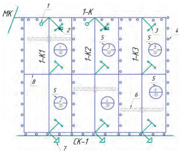
Рис. 3.17. Оросительная сеть на шестипольном севооборотном участке при поливе ЭДМФ «Кубань-Л»: 1 – водовыпуск; 2 – вододеливатель; 3 – трубочатый переезд; 4 – лесополосы; 1-6 – № поля и площадь брутто, га; 6 – ЭДМФ «Кубань-Л»; 7 – концевой сброс; 8 – дорога; МК – магистральный канал; 1-К – севооборотный канал; 1-К1-1-К3 – участковые каналы; СК-1 – сбросный канал
