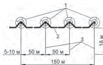
Рис. 9.13. Схема передвижного поливного комплекта ППК-25:
