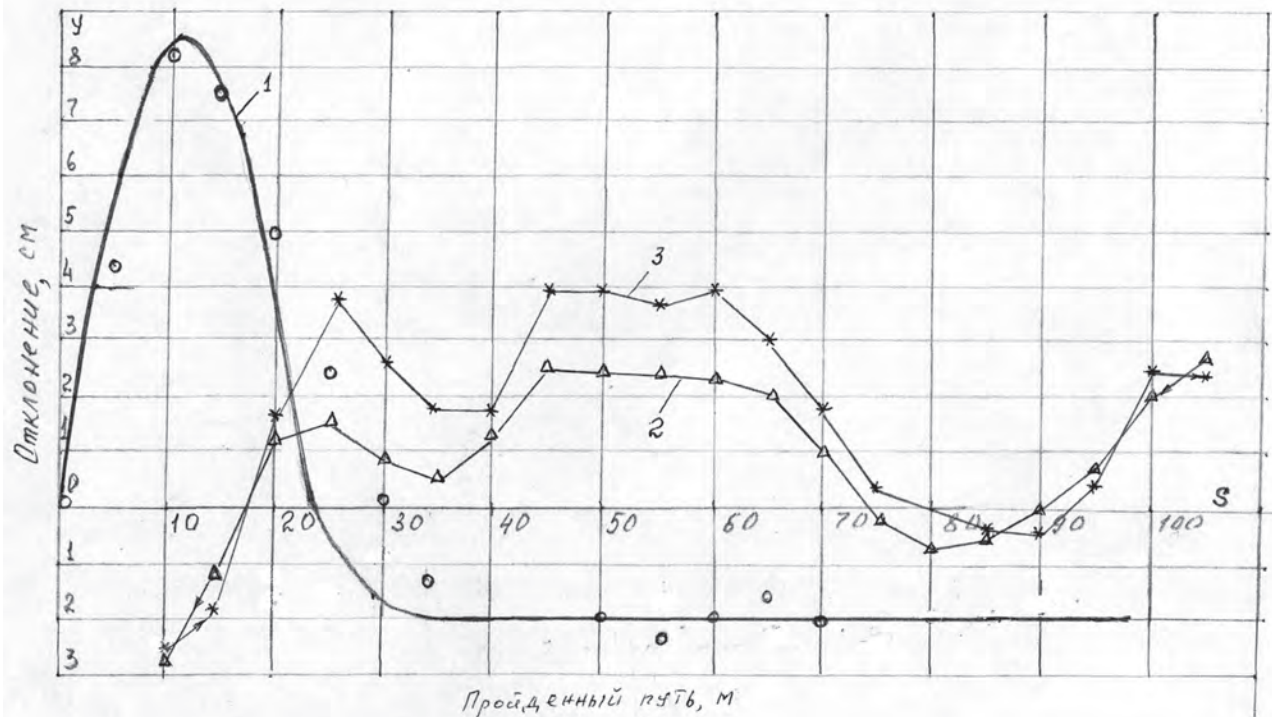
Рис. 3.31. Траектория движения центральной тележки ФДМ «Кубань-Л» по орошаемому участку с системой управления: 1 – теоретическая траектория движения центральной тележки машины при начальной ее установке под углом \varphi=0,92^\circ и о – фактическое значение; 2, 3 – экспериментальные отклонения центральной тележки машины при неоднократном движении машины и образовавшей колеи соответственно от начала к концу поля (кривая 2, \Delta – фактическое значение) и обратном направлении (кривая 3, * – фактическое значение) от возмущающих воздействий y_e
