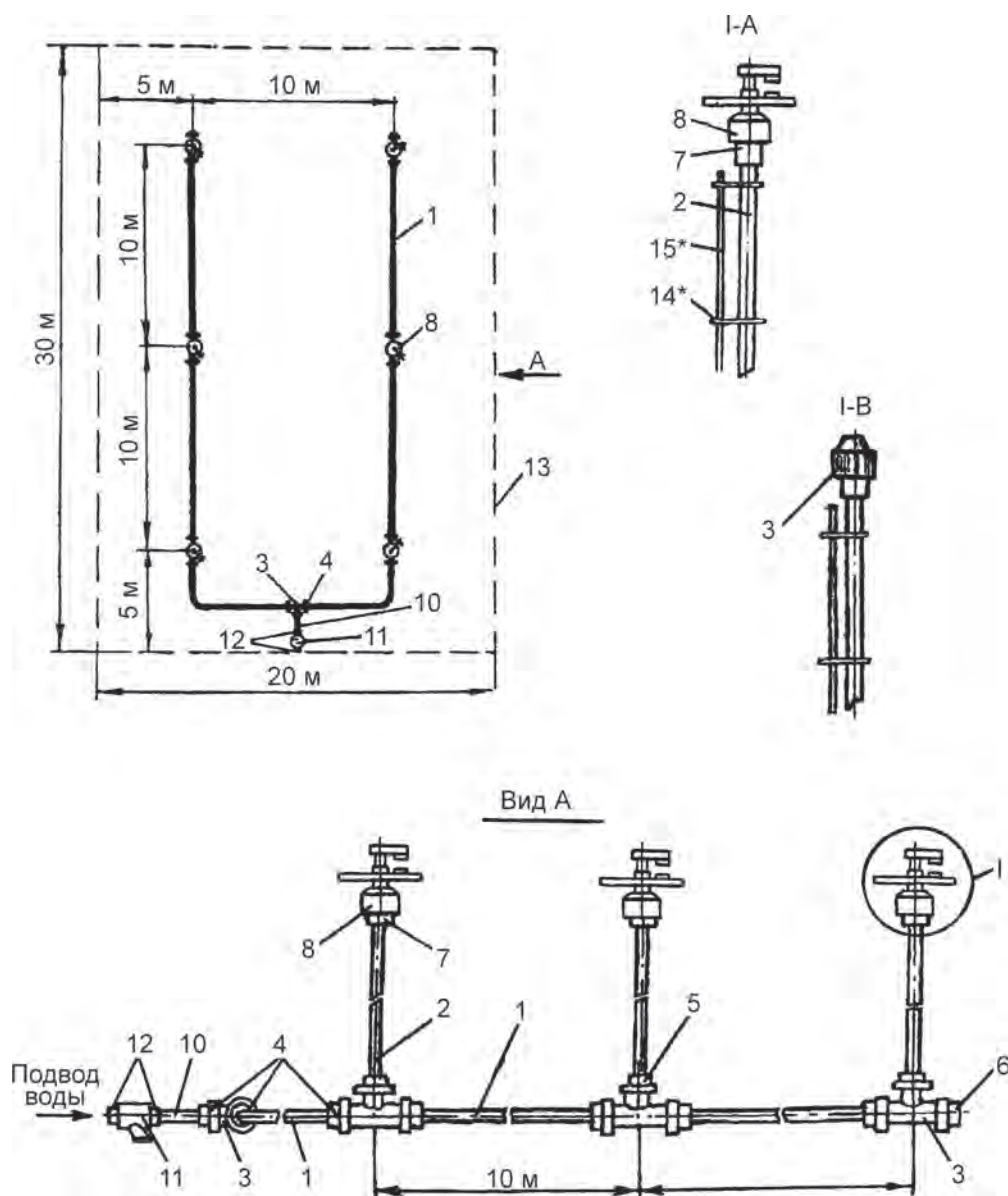
Рис. 7.12. Схема расположения оборудования: 1 – распределительный трубопровод ПНД-20; 2 – поливной трубопровод (стояк) ПВД-16; 3 – тройник; 4 – муфта МЗ6х20; 5 – муфта МЗ6х16; 6 – муфта-заглушка МЗ6; 7 – штуцер G1/2"; 8 – малорасходный дождевальная аппарат (МДА); 9 – заглушка поливного трубопровода G1/2"; 10 – патрубок подсоединительный ПНД-20; 11 – фильтр ФММ-20; 12 – штуцер G3/4"; 13 – граница модульного участка; 14* – шпигат крепежный; 15* – стойка
