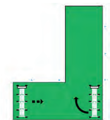
Рис. 3.5. L-образная фронтальная схема движения ЭДМ
