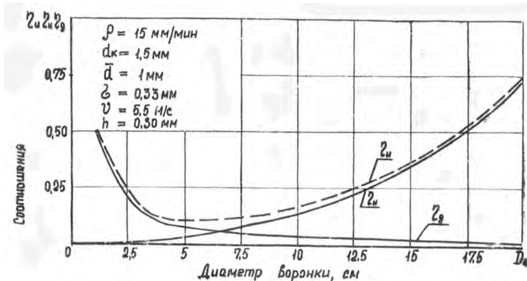
Рис. 1.3. Зависимости раздробленных и «налагаемых» капель от диаметра воронки: \eta_o — раздробленных; \eta_n — «налагаемых»; \eta_u — суммарных
