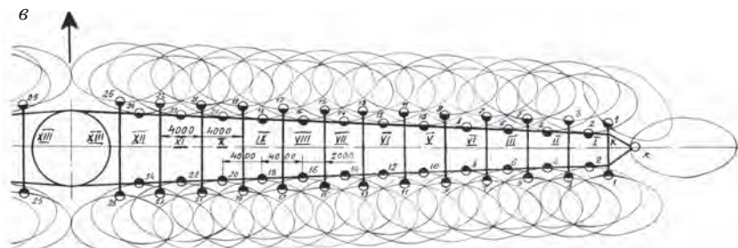
Рис. 3.35. Схемы расстановки дождеобразующих устройств на дождевальном агрегате ДДА-100МА и карты формирования дождя: а – серийный; б – модернизированный для почв средней и пониженной водопроницаемости; в – модернизированный для почв низкой водопроницаемости
