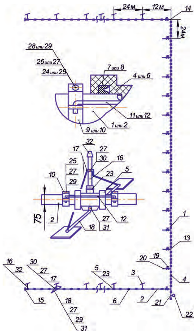
Рис. 5.4. Монтажная схема комплекта КИ-10
