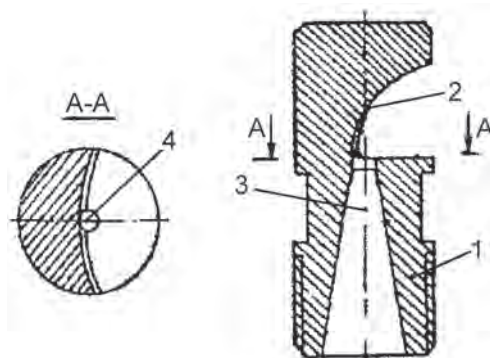
1 – корпус; 2 – сферический дефлектор; 3 – проходной канал в форме конфузора
