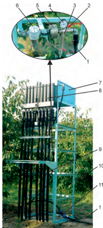
Рис. 8.13. Узел автоматизированного распределения водоподдачи в саду: 1 – подводящий трубопровод; 2 – кран; 3 – фильтр; 4 – манометр; 5 – стабилизатор расхода; 6 – счётчик воды; 7 – ёмкость; 8 – распределитель; 9 – распределительные трубопроводы; 10 – опора; 11 – опорная плита
