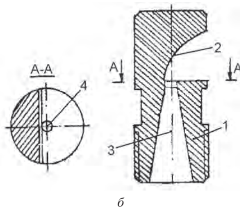
1 – корпус; 2 – цилиндрический дефлектор; 3 – проходной канал в форме конфузора
