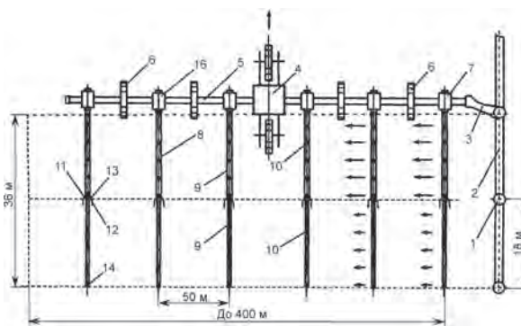
Рис. 9.14. Трубопровод колесный поливной ТКП-ППР:
