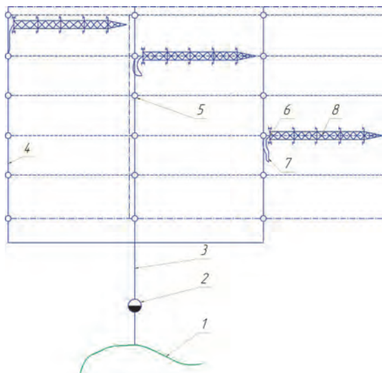
Рис. 3.14. Схема оросительной системы с дождевальной шланговой машиной «Ладога»: 1 – водоисточник; 2 – насосная станция; 3 – магистральный трубопровод; 4 – распределительный трубопровод; 5 – гидрант; 6 – энергетическая тележка; 7 – шланг подключения к гидранту; 8 – дождевальная машина
