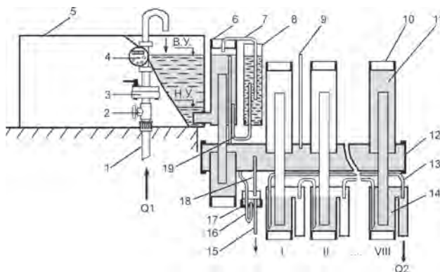
Рис. 8.15. Принципиальная гидравлическая схема сифонного узла автоматического распределения водоподачи:
