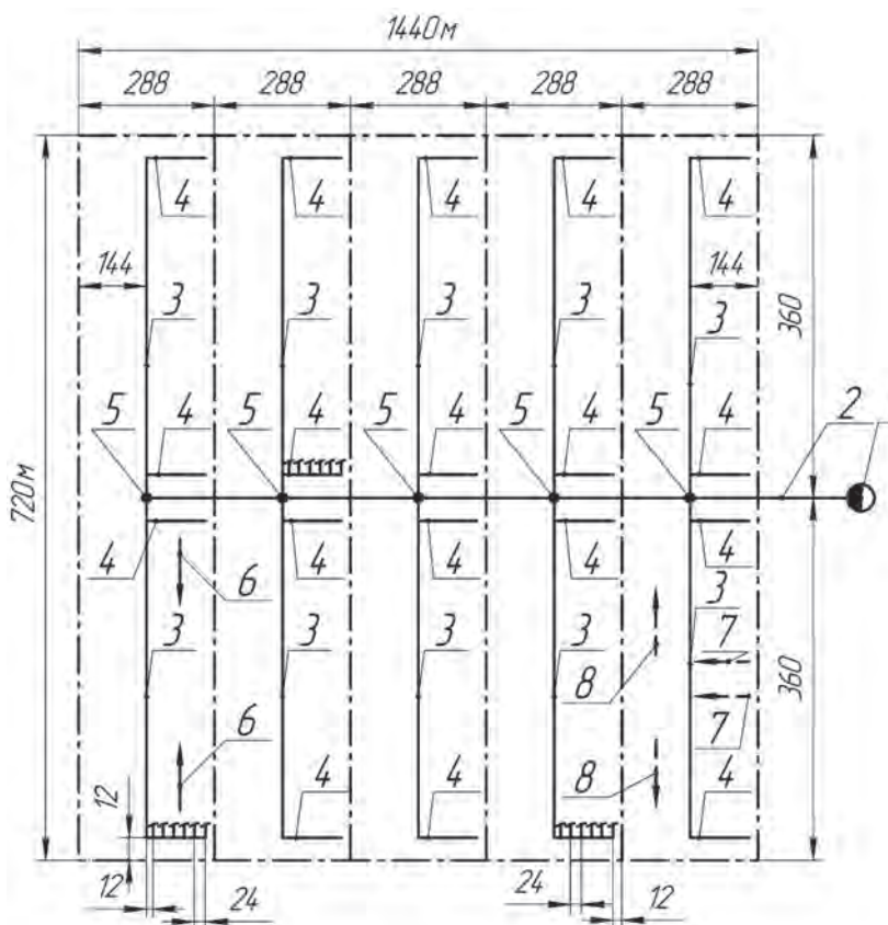
Рис. 5.20. Схема орошения участка десяти комплектами КИ-10 ( S=103,68 га, расход 100-110 л/с): 1 – насосная станция; 2 – магистральный трубопровод закрытой оросительной сети; 3 – распределительный трубопровод \varnothing 110 мм, l = 348 м комплекта КИ-10; 4 – дождевальное крыло \varnothing 75 мм, l = 132 м; 5 – гидрант с узлом подсоединения распределительных трубопроводов двух комплектов КИ-10; 6, 7, 8 – направления перемещения дождевальных крыльев
