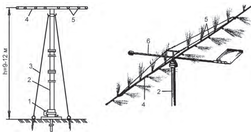
Рис. 6.17. Схема мелкодисперсной стационарной установки ВНИИ «Радуга»: 1 – основание стойки; 2 – стойка; 3 – растяжки; 4 – штанга поворотная; 5 – форсунки; 6 – флюгер
