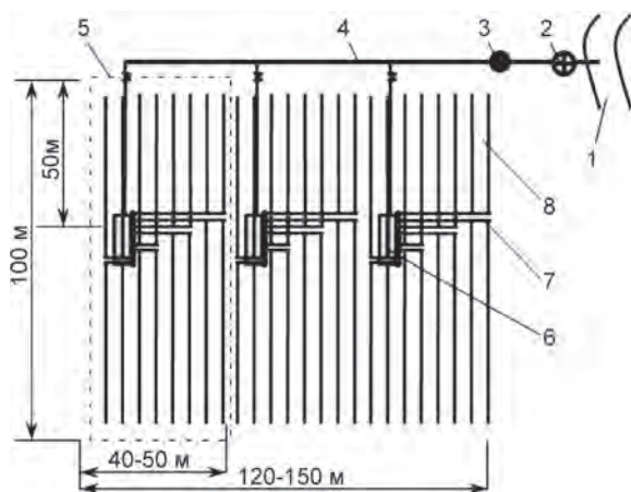
Рис. 8.11. Схема МИЛОС-М-1,0 на площади 1 га: 1 – водопитатель; 2 – насосная станция; 3 – гидроподкормщик; 4 – напорный трубопровод; 5 – блок МИЛОС-М; 6 – накопительно-распределительный узел; 7 – распределительный трубопровод; 8 – поливной трубопровод
