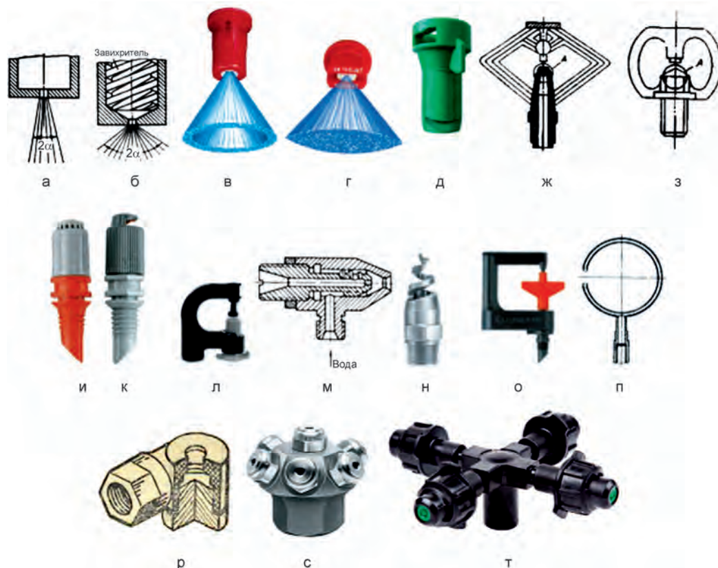
Рис. 6.16. Типы форсунок: а – струйная ( 2\alpha = 10 - 15^\circ ); б – центробежная с завихрителем ( 2\alpha = 50 - 110^\circ ); в – струйная с полым коническим факелом; г – струйная с плоским факелом; д – струйная с боковым факелом; ж, з, и, к, л – струйные с отражающим дефлектором; м – центробежная с завихрителем и подсосом воздуха; н – струйная с завихрителем; о – с разбрасывающим диском; п – струйная с соударяющимися струями; р – тангенциальная; с, т – фоггер (блок насадок)
