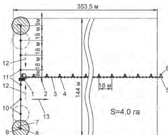
Рис. 4.5. Схема полива участка шланговым дождевателем с комплектом разборного трубопровода Ø75 мм: 1 – шланговый дождеватель; 2 – полиэтиленовая труба, l = 6 м, Ø 75 мм; 3 – муфта Ø75 мм; 4 – тройник с вентилем Ду 65; 5 – входной патрубок; 6 – манометр; 7 – трубопровод дождевателя; 8 – дождевальный аппарат (Д.А.) на опоре; 9, 10, 11 – позиции Д.А. при поливе; 12 – направление перемещения аппарата; 13 – направление перемещения шлангового дождевателя вдоль трубопровода
