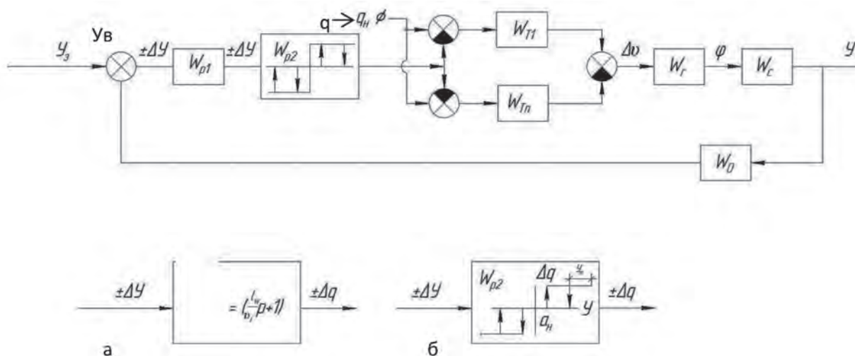
Рис. 3.30. Структурная схема системы управления фронтальной машины «Кубань-Л» с обратной связью: а – регулирующее звено по производной в обратной цепи W_o ; б – нелинейное форсирующее звено W_{p2} ; W_{p1} – линейное (пропорциональное) звено; W_r , W_r , W_c – динамические звенья опорной тележки, разворота и смещения машины соответственно; y_3 , y , y_o – заданное, текущее и возмущающее смещение машины; y_o – величина снижения отклонения машины от максимального; a_n – порог чувствительности регулятора; \phi – угол поворота машины
