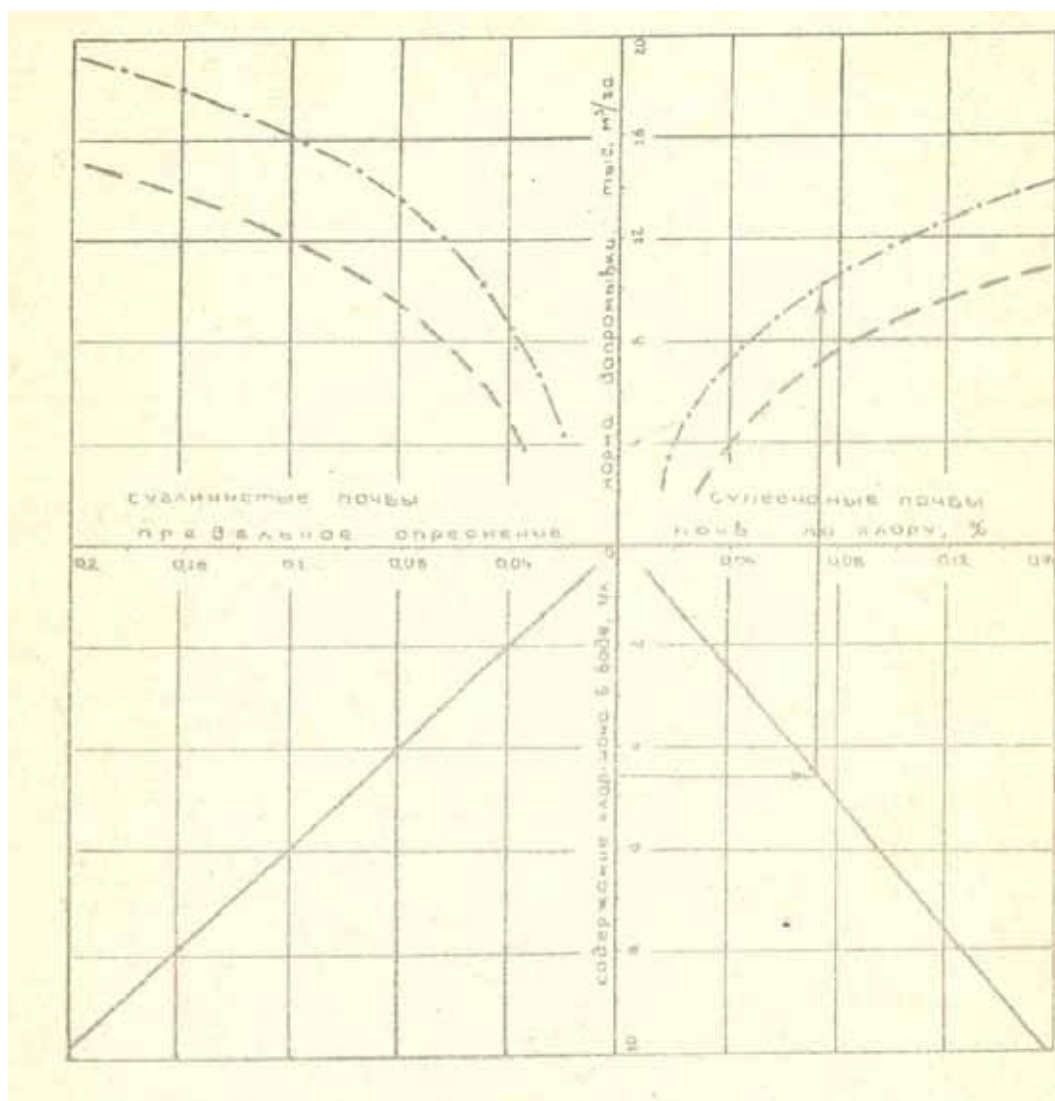
Рис.4 Номограмма для расчета норм допрымывки почв по хлор иону; — · — · — до 0,01% ; — — — до 0,02%.
