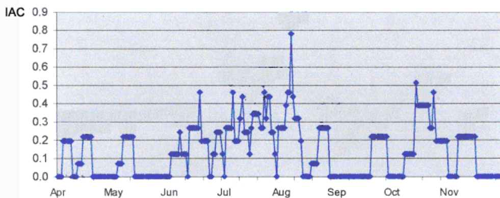
Рис. 4. Суточная динамика коэффициента «покрытия» орошаемой площади поливами (IAC) для участка дренируемого дренажом - УД-3 (2001)
