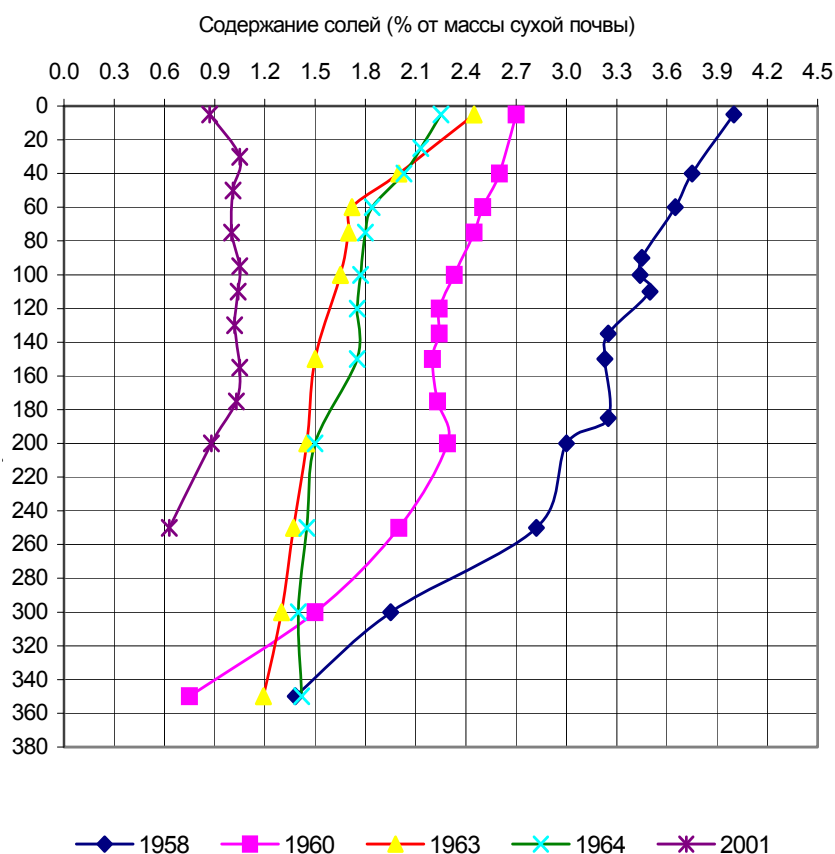
Рис. 5. Изменение содержания солей в почвогрунтах
