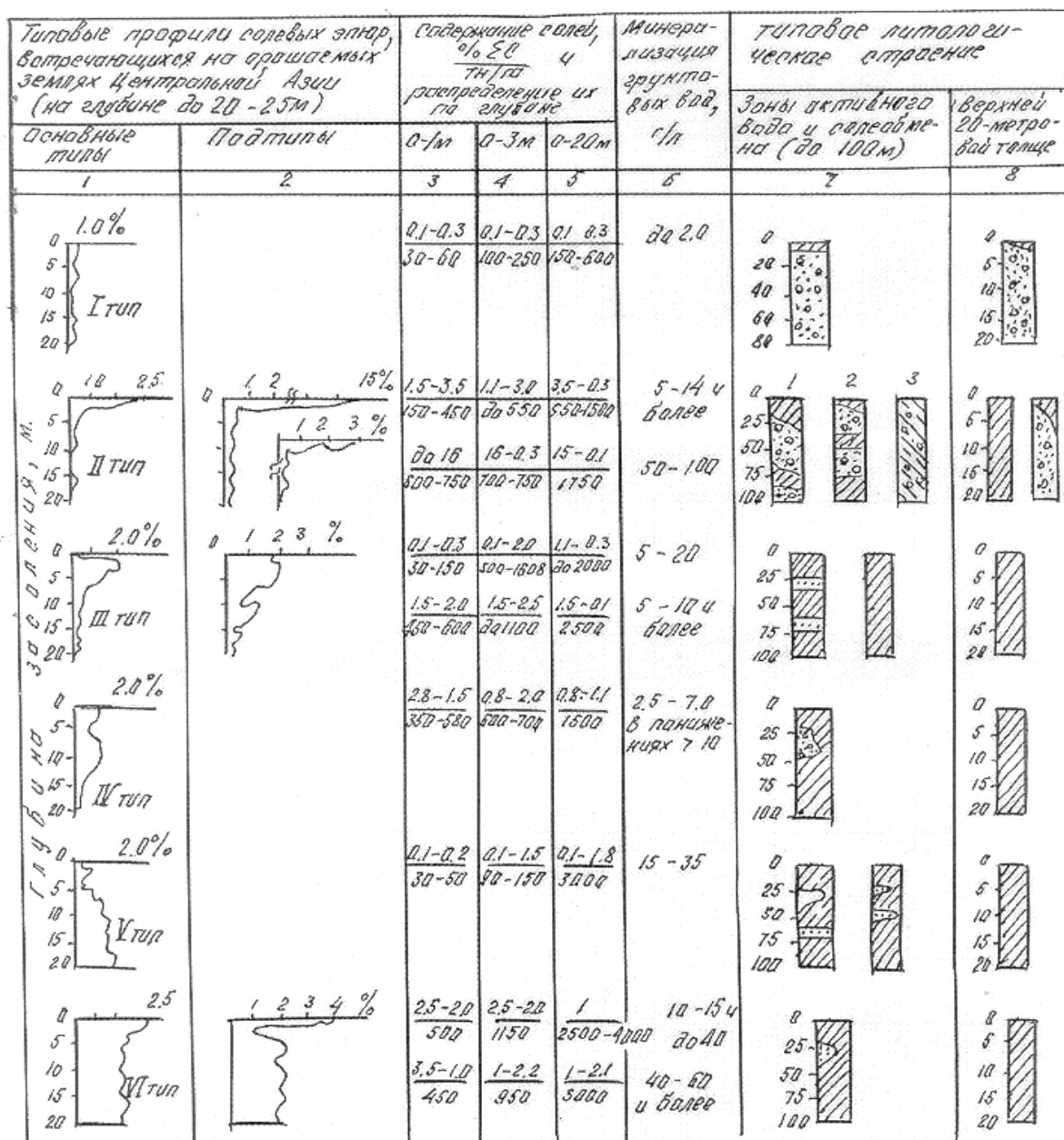
Рис. 2. Типы солевых профилей на орошаемых землях Центральной Азии (В.А. Духовный и др., 2004)
