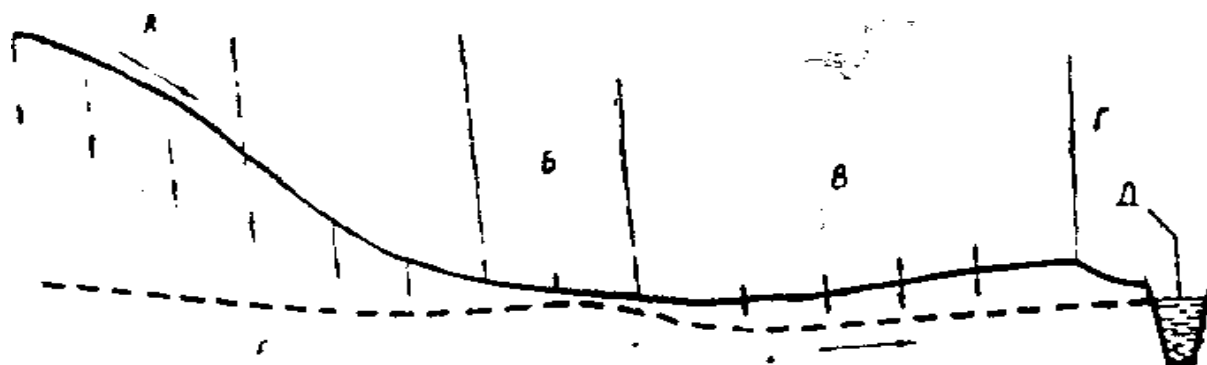
Рис .1. Схема гидрогеологических зон территории Центральной Азии: А - зона погружения поверхностных вод; Б - зона выклинивания грунтовых вод; В – зона рассеивания грунтовых вод; Г - пойма реки; Д – река.
