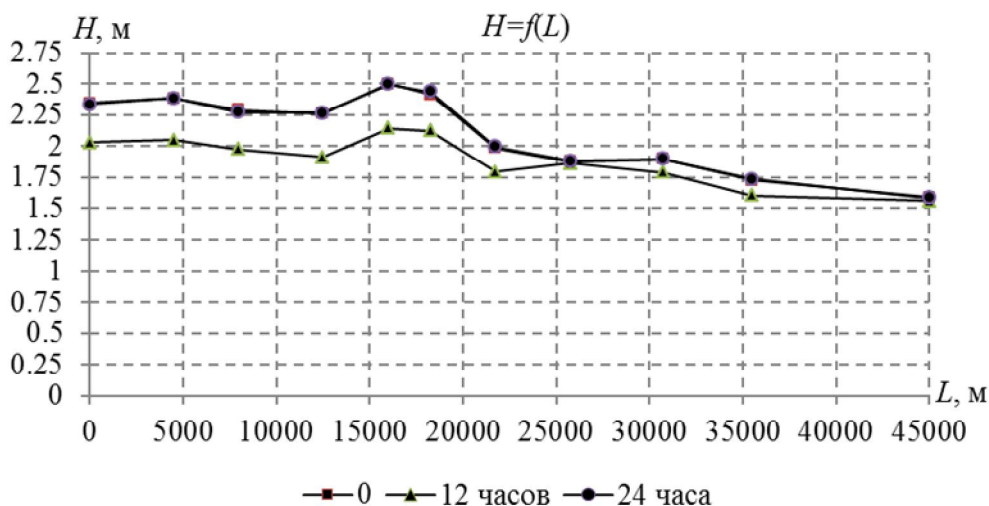
Рисунок 1 – Зависимость изменения глубин воды от удаленности бьефов от головного створа магистрального канала для отбора расходов воды 98 % обеспеченности при наличии регуляторов уровней по нижнему и верхнему бьефам сооружений (регулирование с перетекающими объемами)
