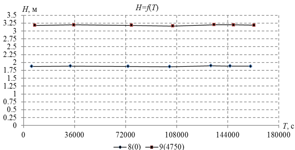
Рисунок 3 – Зависимость изменения уровней от времени в начальном створе 8-го и конечном створе 9-го бьефов для отбора расходов воды 98 % обеспеченности при наличии регуляторов уровней по нижнему и верхнему бьефам сооружений (регулирование с перетекающими объемами)
