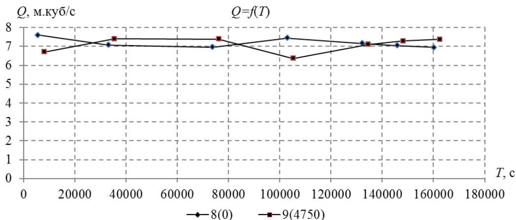
Рисунок 4 – Зависимость изменения расходов от времени в начальном створе 8-го и конечном створе 9-го бьефов для отбора расходов воды 98 % обеспеченности при наличии регуляторов уровней по нижнему и верхнему бьефам сооружений (регулирование с перетекающими объемами)
