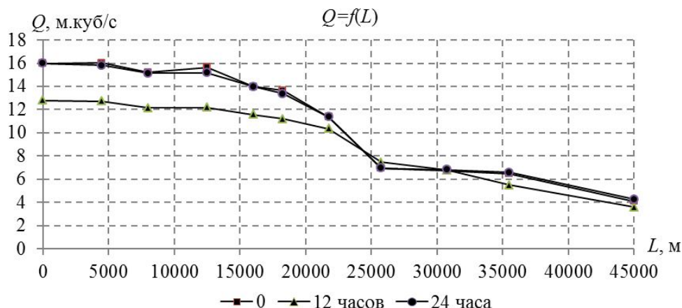
Рисунок 2 – Зависимость изменения расходов воды от удаленности бьефов от головного створа магистрального канала для отбора расходов воды 98 % обеспеченности при наличии регуляторов уровней по нижнему и верхнему бьефам сооружений (регулирование с перетекающими объемами)
