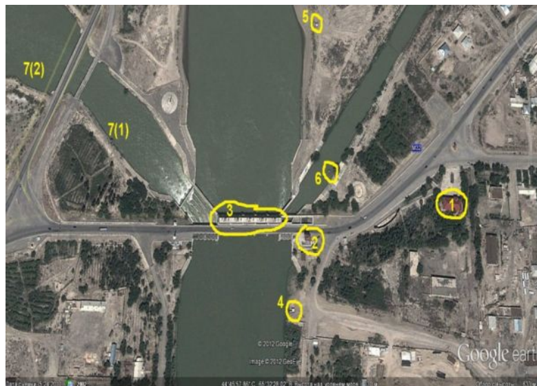
Рис. 1. План установок автоматизированных технических средств контроля: 1- диспетчерская; 2- шкаф с контроллером; 3- плотина. 4- ультразвуковой датчик уровня воды верхнего бьефа; 5-датчик уровня воды нижнего бьефа; 6-ультразвуковой датчик правобережного канала; 7- датчик уровня левого канала, устанавливаемый в позиции 7(1) или в позиции 7(2).
