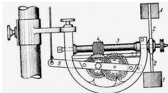
Рис. 1. Механический счетчик Рейгарда Вольмана (по [2])
