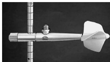
Рис. 6. Малый ИСП С2 и преобразователь сигналов Z-215 (ОТТ-Hydrometrie, г. Кемптен, Германия) (по [18])
