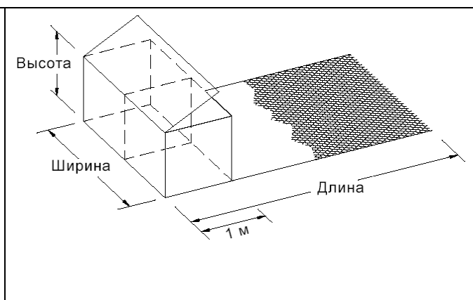
Рис. 3. Система Террамеш
