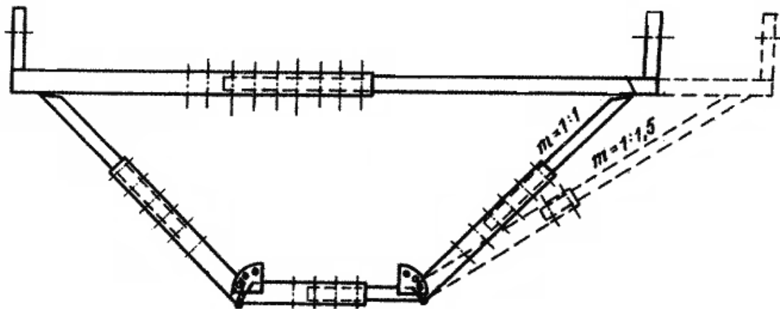
Рисунок 3 – Несущая рама устройства для укладки бетонной облицовки каналов (УкрНИИГиМ) [7]
