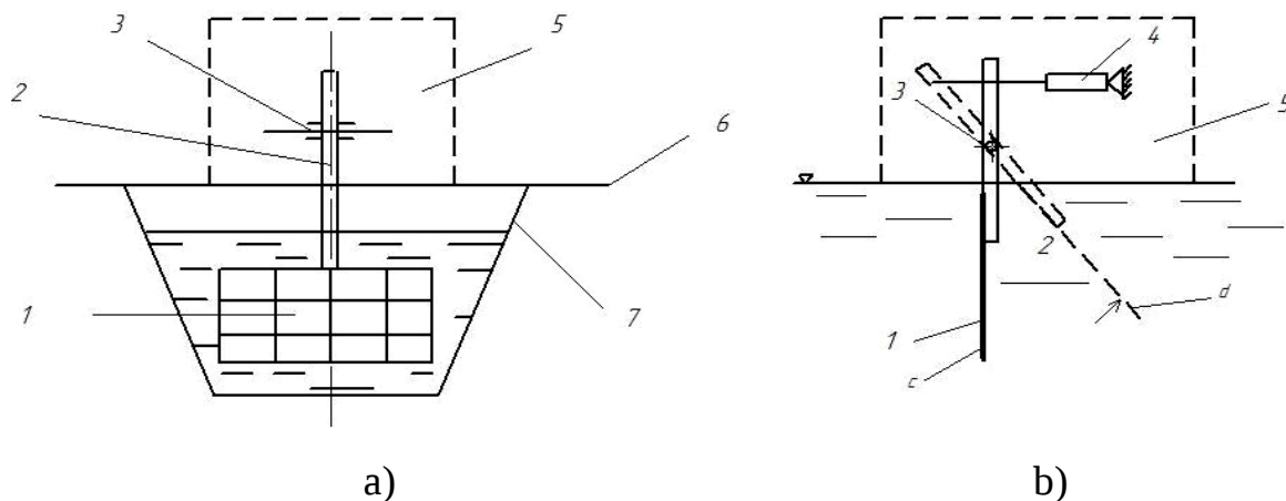
а – общий вид расположения расходомера на канале; б – принципиальная схема работы; с – первоначальное положение; d – рабочее положение; 1 – чувствительный элемент; 2 – нижняя часть рычага; 3 – ось вращения; 4 – пружинный динамометр; 5 – защитный короб; 6 – гидрометрический мостик; 7 – канал
