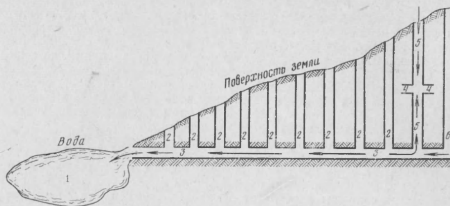
План оросительного канала (кяриза): 1 — жалава (наземный колодец); 2 — дикана (колодцы); 3 — отук (сөө) — (тоннель); 4 — сувалы гатлак (водоносный пласт); 5 — колодец, вырытый способом дубул; 6 — пешкар (головной колодец)
