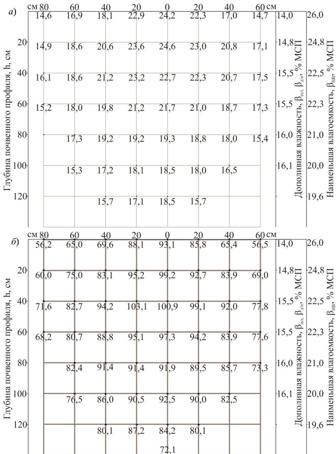
Рисунок 1 – Матрицы данных измерений влажности почвы в подкапельном почвенном пространстве
