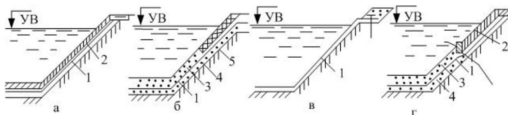
а – бетонопленочные; б – грунтопленочные; в – поверхностные; г – комбинированные; 1 – полимерный противofильтрационный экран; 2 – бетонное покрытие; 3 – защитный слой грунта; 4 – подстилающий слой; 5 – крепление защитного слоя
