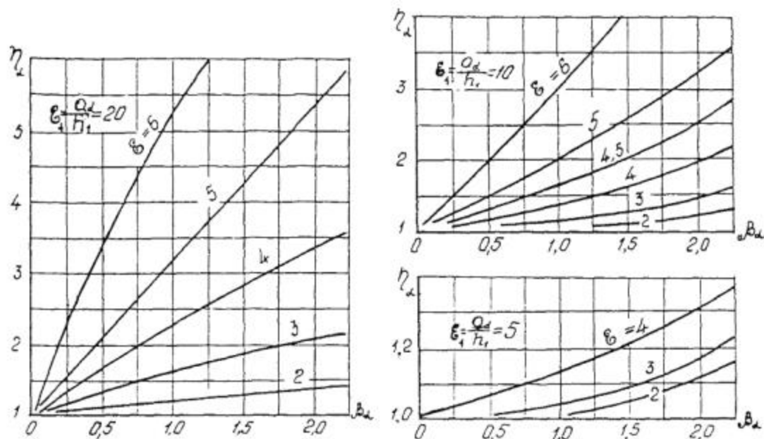
Черт. 8.11. Графики для определения коэффициента h_a
