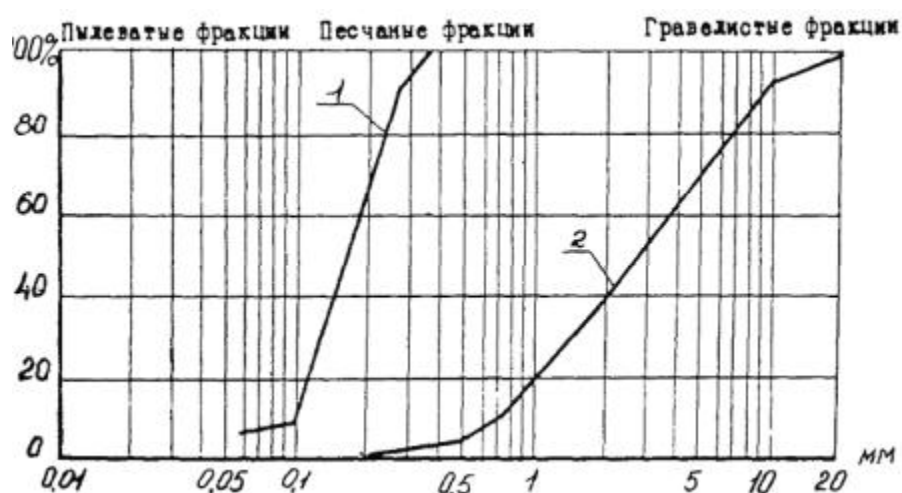
Черт. 7.2. Кривые предельного гранулометрического состава обсыпок для дрена с фильтрами из волокнистых материалов:
