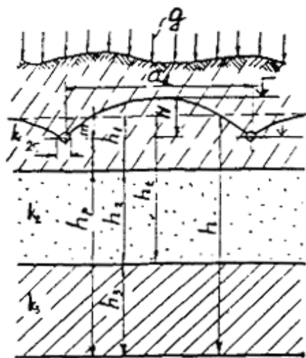
Черт. 8.5. Расчетная схема двухслойной толщи при расположении дренажа и свободной поверхности подземных вод в нижнем слое
