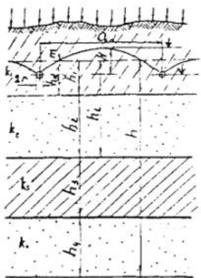
Черт. 8.9. Расчетная схема четырехслойной толщи с дренажем в верхнем слое
