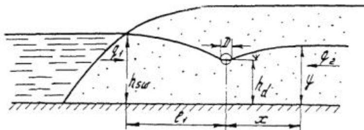
Черт. 9.2. Схема для расчета береговых дрены
