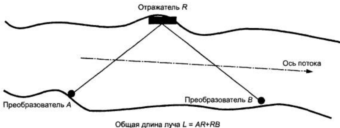
Рисунок 2 - Схема расположения преобразователей с отражением лучей
