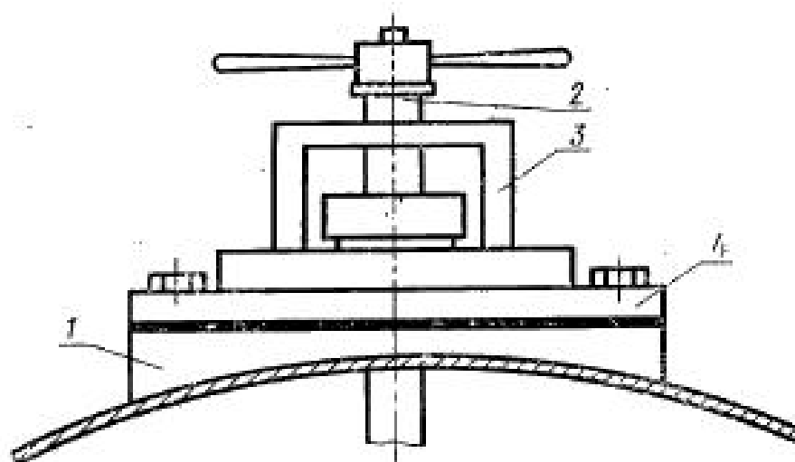
1 — закладка; 2 — штанга первичного преобразователя скорости; 3 — калибровочный ввод; 4 — фланец
