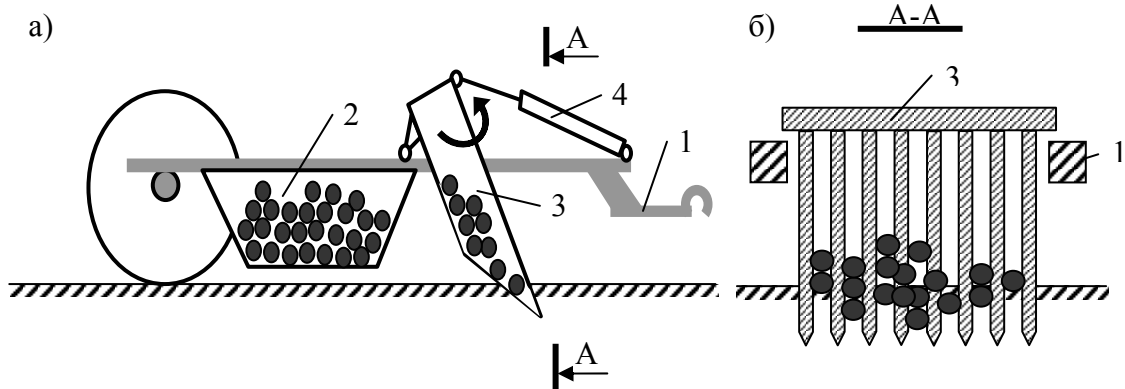
Рис. 1.1.1. Универсальный камнеподборщик УКП-0.6. ( d_k=12...65 см):
