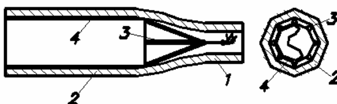
Рис. 4.6.1. Сохранение пропускной способности трубопровода: 1 - старая труба; 2 - старая труба после расширения; 3 – ломающий трубу расширитель
