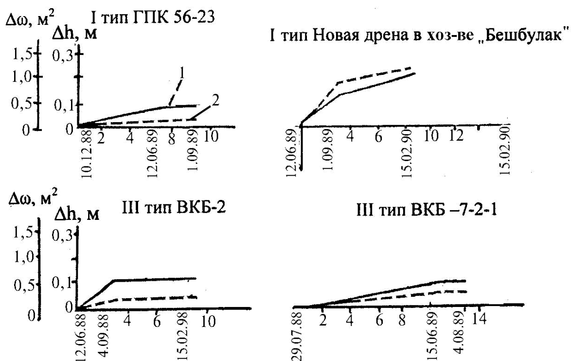
Рис.21. Интенсивность заилиения дрена (Гаипназаров, 1987 г). 1 – толщина h , м; 2 – площадь \Delta w , м 2 .
