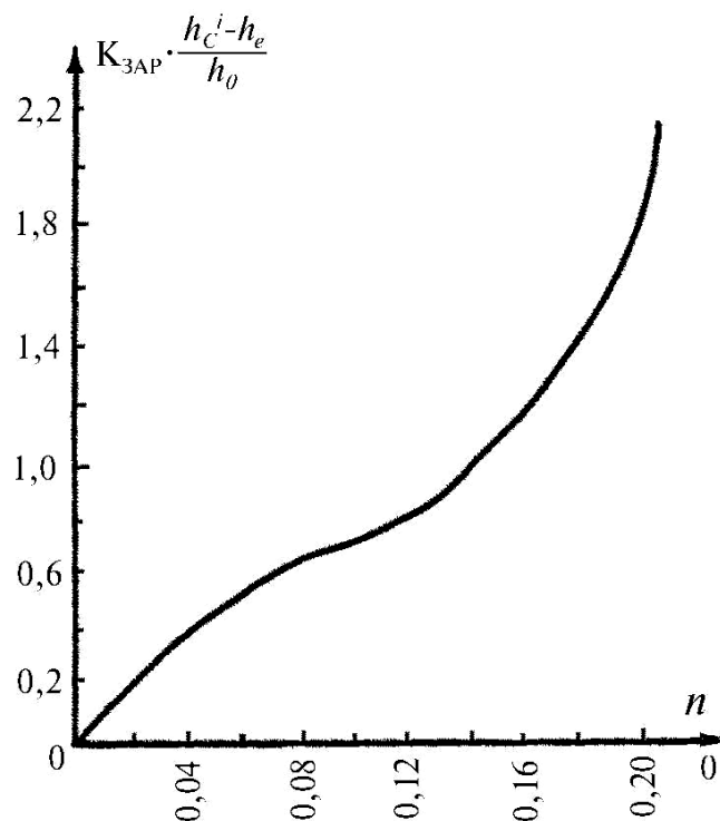
Рис.28. График зависимости наполнения открытой КДС от изменения её шероховатости (Гаипназаров, 1987 г).
