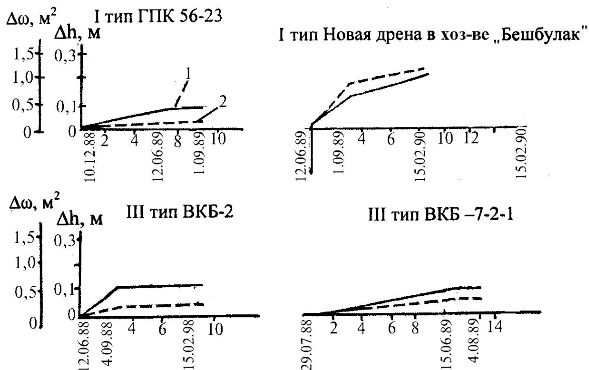
Рис.5.4. Интенсивность заилиения дрен (Гаиппазаров, 1987 г). 1 – толщина h , м; 2 – площадь \Delta\omega , м².
