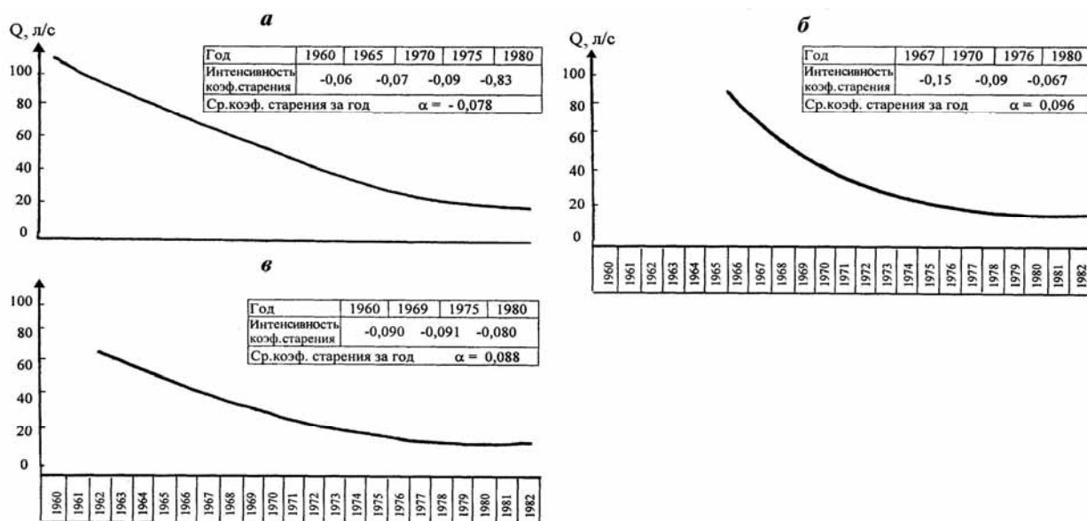
Рис.5.2. Изменение дебита скважин в процессе физико-химического кольтматажа в зависимости от продолжительности их работы при: а – карбонатизации; б – коррозионных явлениях; в – смешанных процессах (Якубов, Джалилова, 1983)
