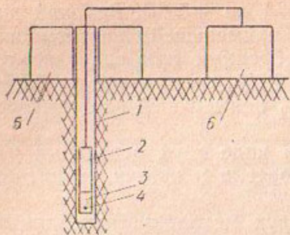
Рис. 1. Блок-схема прибора НИВ-2:
