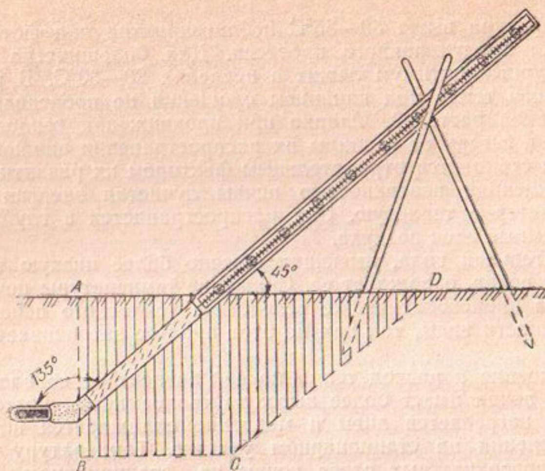
Рис. 2. Термометр Н. И. Саввинова.
