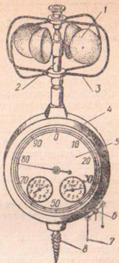
Рис. 3. Ручной анемометр:
