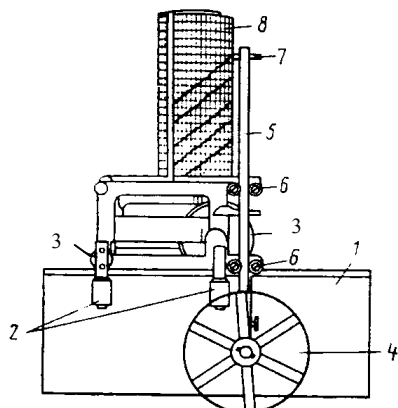
Рис. 6.9. Профилограф для снятия поперечных профилей дороги: 1 – доска; 2 – ролики вертикальные; 3 – ролики горизонтальные; 4 – рабочее колесо; 5 – рейка; 6 – направляющие ролики; 7 – пишущее устройство; 8 – барабан.
