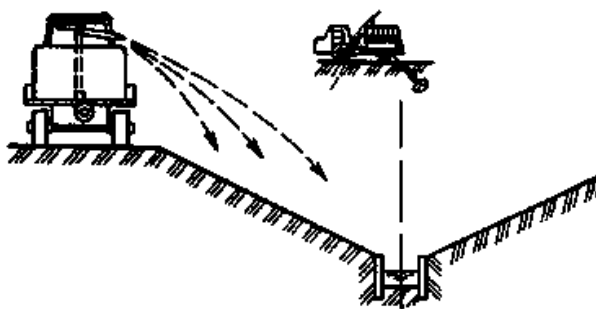
Рис. 4. 25. Нанесение на откос растительной гидросмеси.
