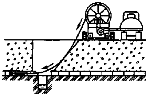
Рис. 4.18. Промывка дренажей и коллекторов от наносов дренопромывочной машиной (Д-910, ПДТ-125 и др.).
