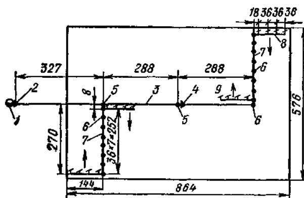
Рис. 5.9. Примерная схема при поливе установкой КИ-50 “Раду-га”: 1 – насосная станция; 2, 4 – переходники 180×150; 3, 7 – магистральный и распределительный трубопроводы; 5, 6 – трубы-гидранты диаметром 150 и 125 мм; 8, 9 – дождевательные крыло и аппарат (размеры в м).
