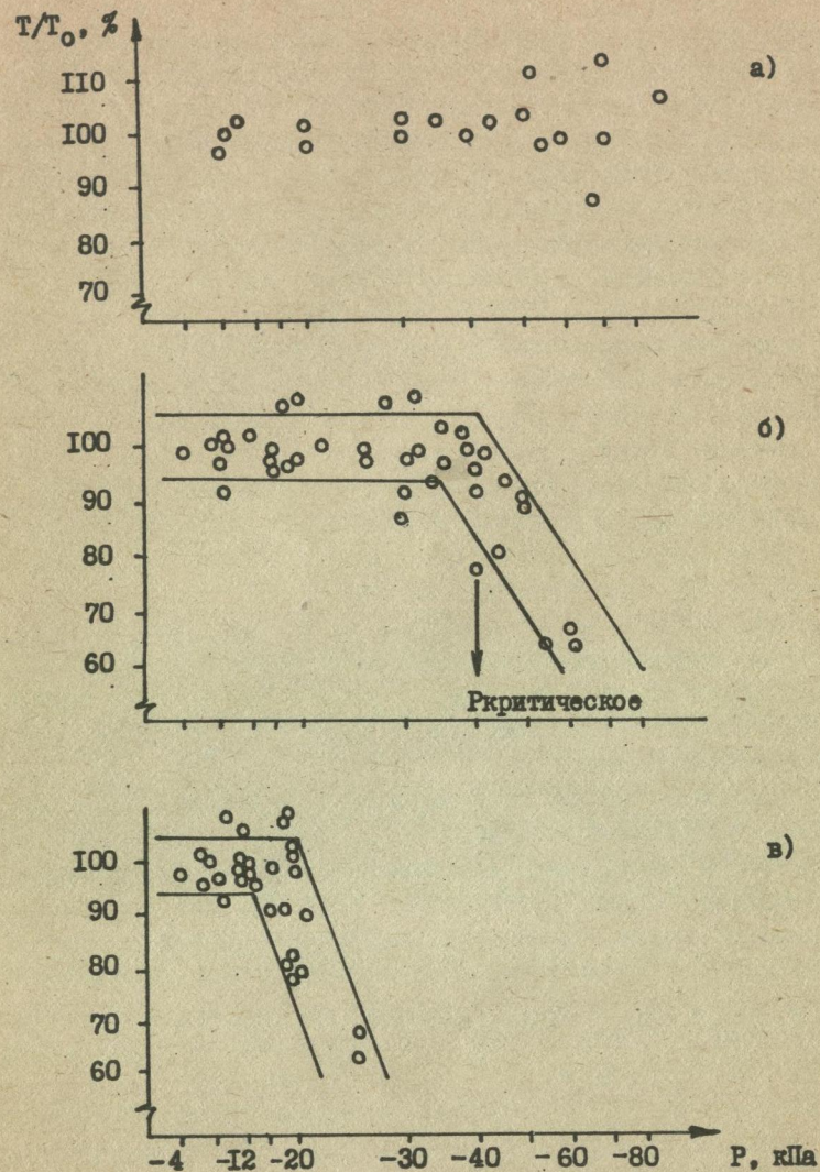
Рис. 2 Зависимость относительной транспирации хлопчатника ( T/T_0 ) от давления влаги (Р, кПа) на глубинах 30 см (а), 40 см (б) и 50 см (в).
