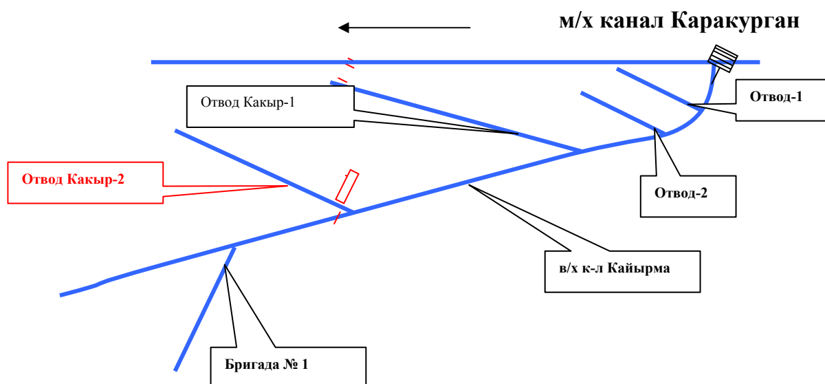
Рис. 1.1.1.2 Прямолинейная схема канала Кайырма АВП «Кызыр-Абад» в Араванском районе.
