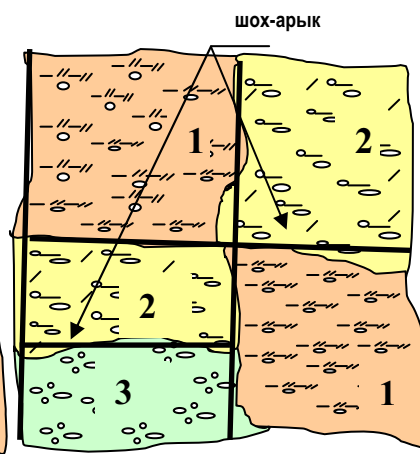
Рис. 7.3 Выделение границ почвенных разностей на поливном поле 1 – средние суглинки с покровным мелкоземом мощностью более 1 метра; 2 – легкие маломощные суглинки, подстилающиеся галечником; 3 – вскрытый галечник, заполненный легким суглинком;
