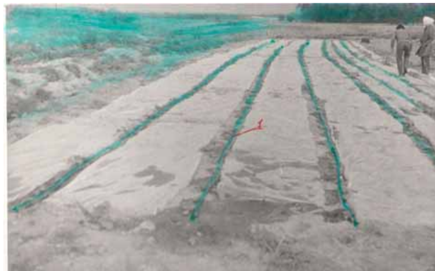
Фото 2 Ручная укладка полиэтиленовой пленки под систему капельного орошения огурцов 1 – поливной трубопровод с капельницами Молдовия-1А
