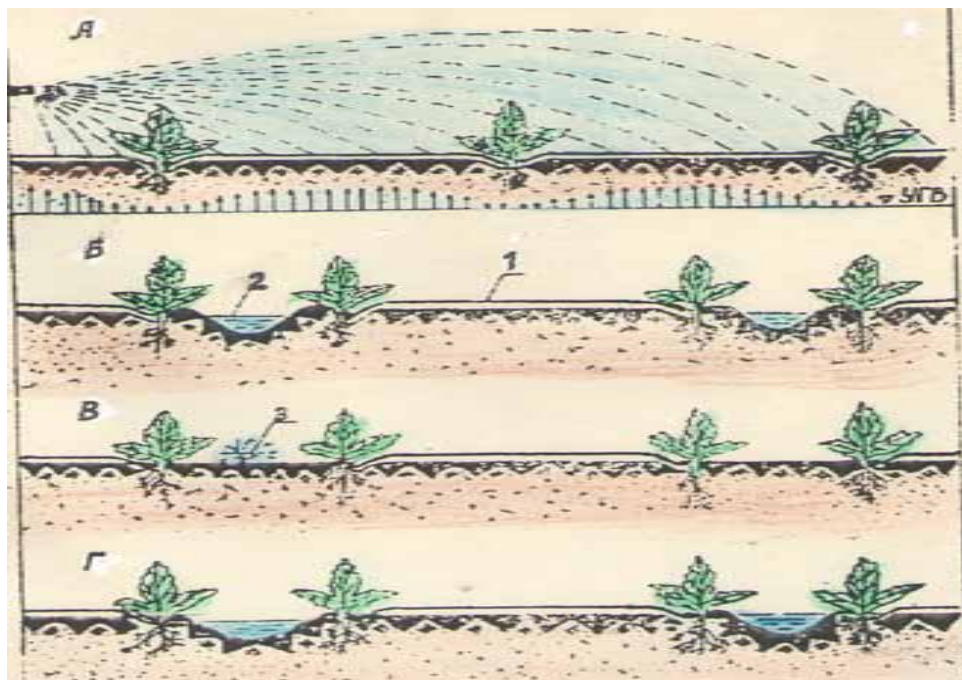
Рис.1 Рекомендуемые схемы мульчирования междурядьев прозрачной полиэтиленовой пленкой при разных способах полива: А – при субирригации и дождевании; Б – при поливе по бороздам (1 – полиэтиленовая пленка; 2 - борозда); В – при капельном орошении (3 – поливной трубопровод); Г – при посеве семян под засыпанные края пленочной ленты.
