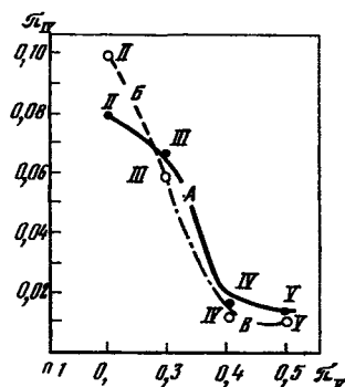
Рис. 25. Поэтапный характер связи между критериями почвенного подобия \Pi_{гv} (показатель интенсивности изменения солепроявления в почве) и \Pi_v (КЗИ)
