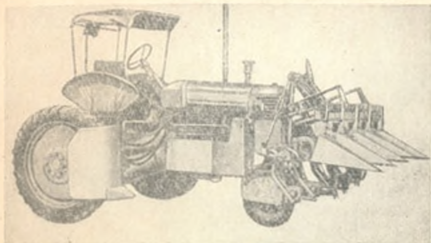
Рис. 17. Приспособление для чековки хлопчатника ЧВХ-4 к культиватору-удобрителю НКУ-4-6А.
