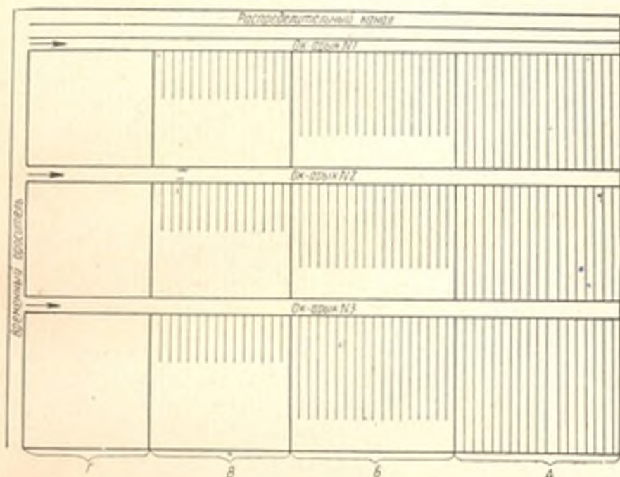
Рис. 6. Схема полива при рядовом посеве хлопчатника.
