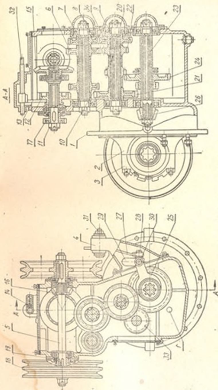
Рис. 26. Раздаточная коробка;
