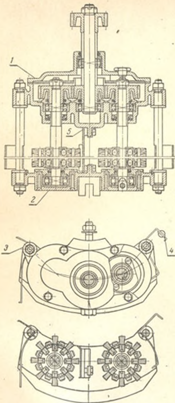
Рис. 24. Щеточный съемник:
