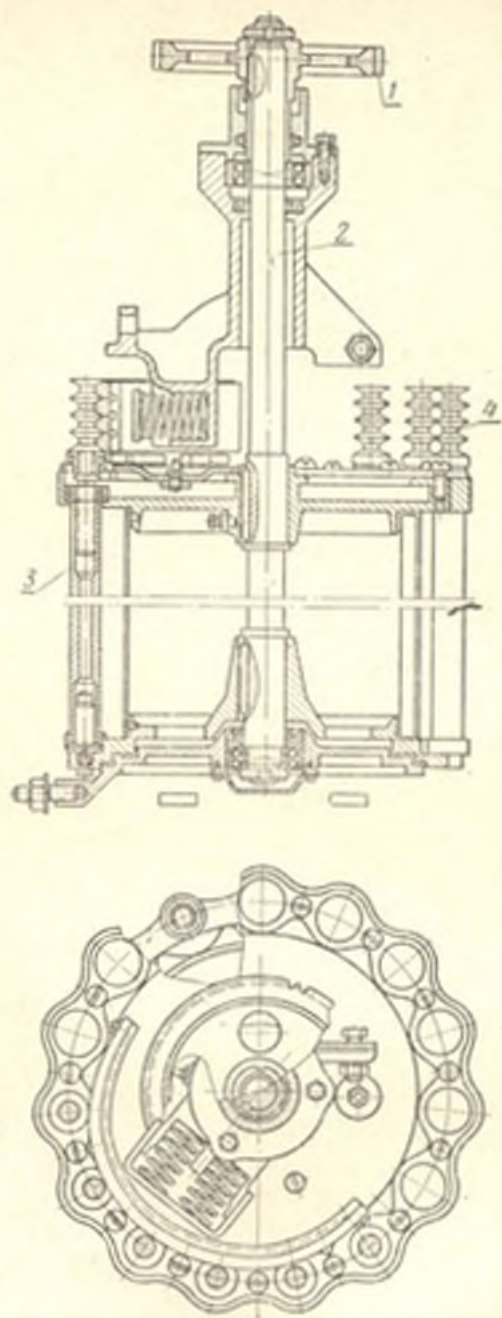
Рис. 22 Шпindelный барабан хлопкоуборочной машины ХВС-1,2: 1 — приводная шестерня; 2 — вал барабана; 3 — шпиндель; 4 — приводные ролики шпинделя.
