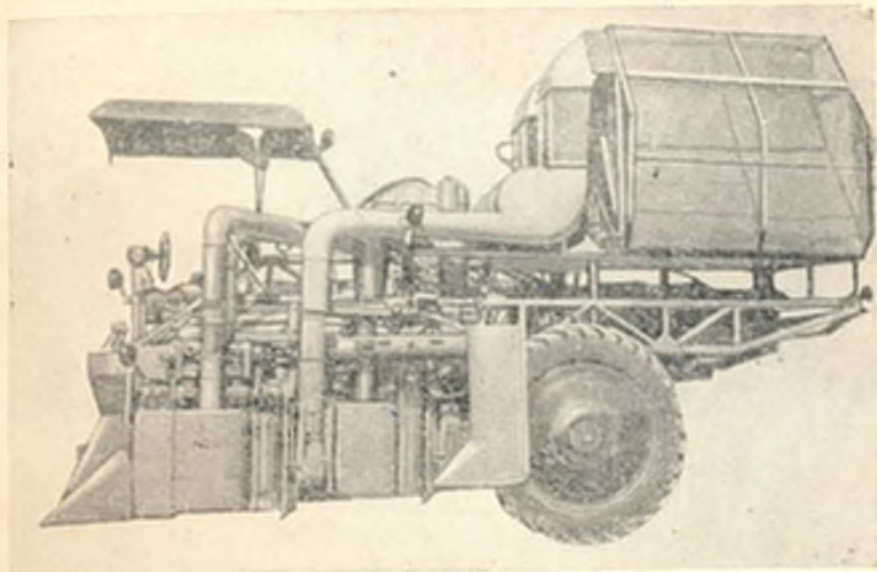
Рис. 21. Хлопкоуборочная машина ХВС-1,2 (общий вид).
