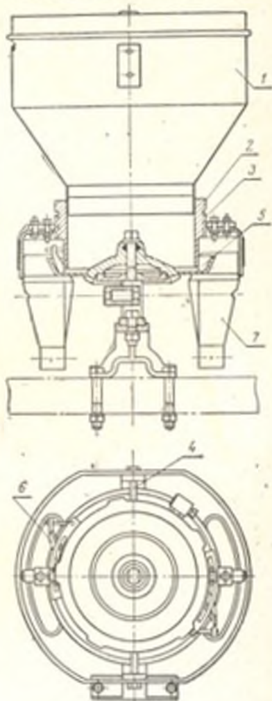
Рис. 16. Культиватор-удобритель НКУ-4-6А:
