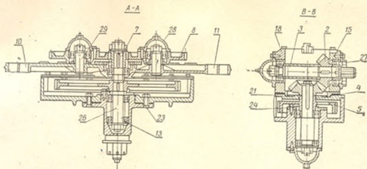
Рис. 25. Распределительная коробка (продолжение).
