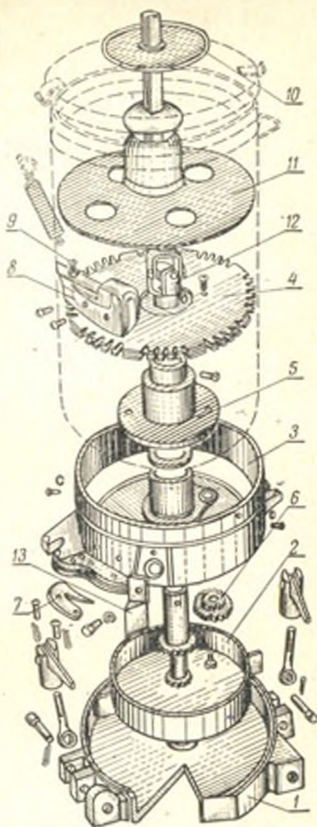
Рис. 10. Высевающий аппарат сеялки СТВХ-4:
