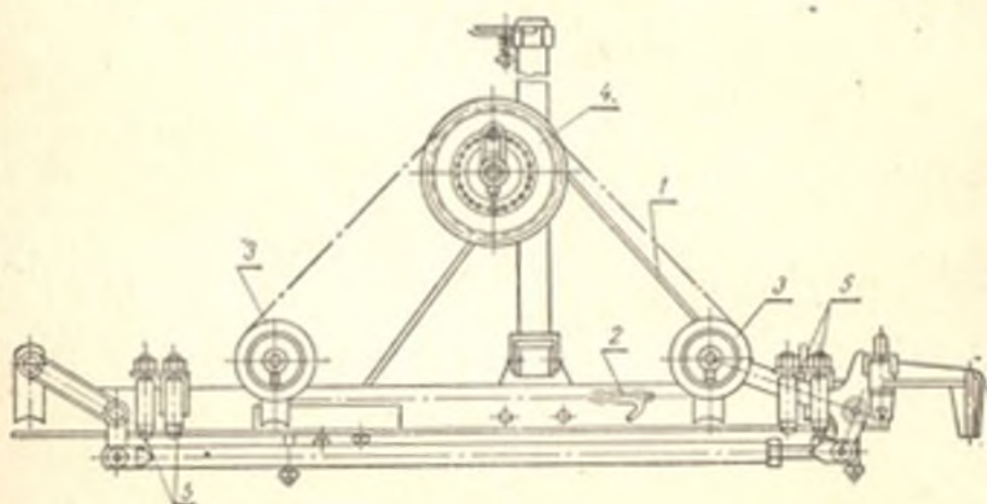
Рис. 13. Привод от мерной проволоки (правый):
