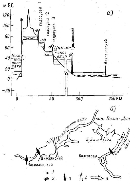
Рис. 12. Продольный профиль (а) и схема (б) трассы переброски части стока р. Волги в р. Дон.
