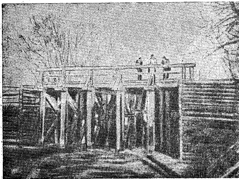
Главное сооружение на протоке Чинили
