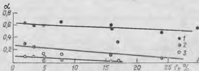
Рис. 2.3. Зависимость коэффициента стока от площади лесов и лесных полос f_{\text{л}} (%) в многоводные (1), средние по водности (2) и маловодные (3) годы для лесостепной и степной зон.
