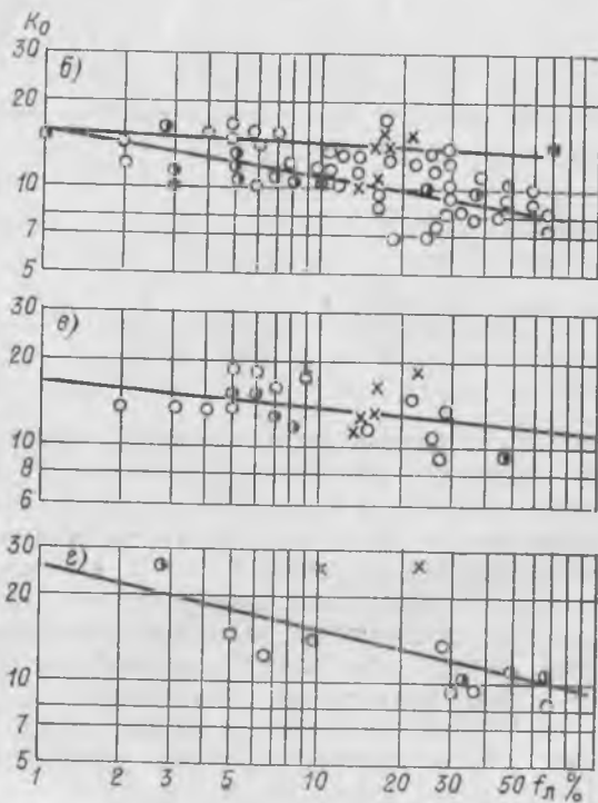
Рис. 4.1. Зависимость K_0 = f(f_l) для прирусловых лесов (1), лесов, расположенных равномерно на водосборе (2) и приводораздельных лесов (3) лесной (а) и лесостепной (б—г) зон.
