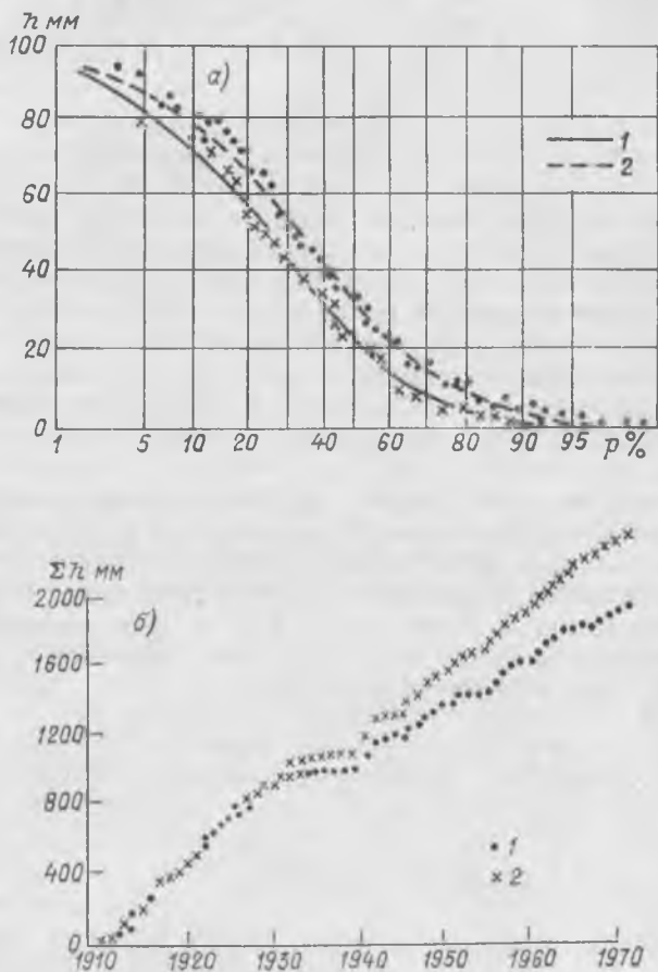
Рис. 2.14. Кривые обеспеченности (а) и интегральные кривые (б) слоя стока весеннего половодья р. Большой Узень у г. Новоузенска за периоды с нарушенным (1) и не нарушенным (2) хозяйственной деятельностью режимом.
