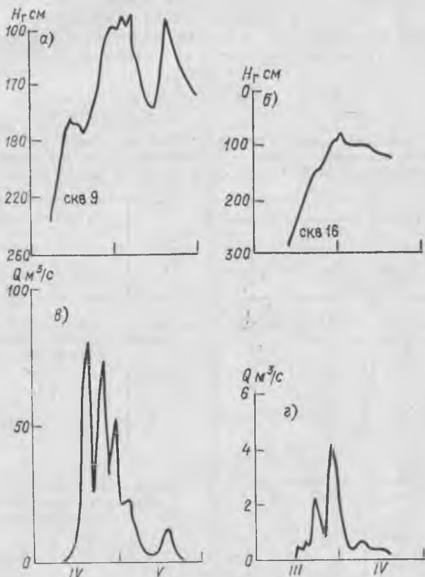
Рис. 2.6. Ход уровня грунтовых вод H_r и стока Q . а, б — лог Усадьевский, ВФ ГГИ (1958 г.); в, г — р. Девица — с. Нижнедевицк (1965 г.).
