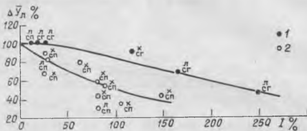
Рис. 2.2. Зависимость от уклона склона уменьшения стока с лесных склонов \Delta u_{\text{л}} (%) относительно безлесных для лесостепной (1) и лесной (2) зон.
