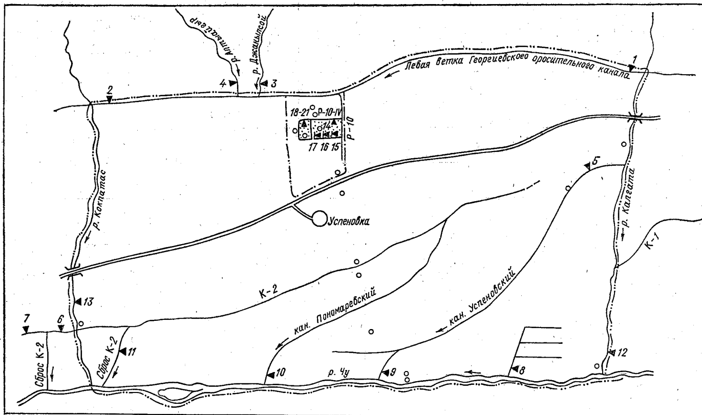
Рис. 5.3. Схема расположения пунктов наблюдений на воднобалансовом участке Георгиевской оросительной системы.
