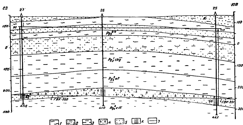
Рис. 2. Поперечный геолого-гидрогеологический разрез через Жаманкоянкуллакское месторождение. 1 — песчаные глины; 2 — глинистые пески; 3 — плотные глины; 4 — газоносные пески; 5 — водоносные пески; 6 — интервалы опробования; 7 — пьезометрическая поверхность подземных вод кумского горизонта.
