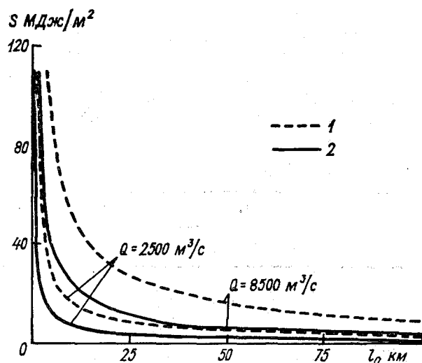
Рис. 7.8. Зависимость положения нулевой изотермы от теплотерь, температуры и расхода воды в период замерзания.
