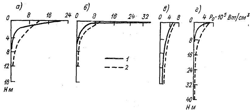
Рис. 7.2. Изменение интенсивности ледообразования по глубине.
