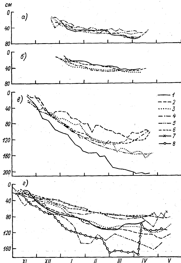
Рис. 4.5. Нарастание толщины льда в различных пунктах по длине реки в течение периода ледостава.
